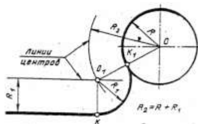
Рис.20 Сопряжения дуги окружности и прямой
