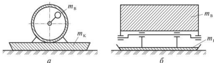
Рис. 6.9. Принципиальные схемы вибротрамбующих машин с центробежным (а) и колебаний (б)
