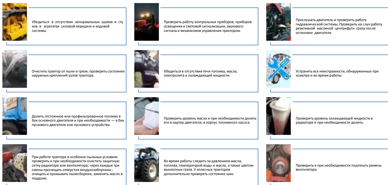
Рисунок 2 – Ежедневный технический уход трактора
