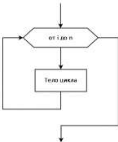
Цикл for
