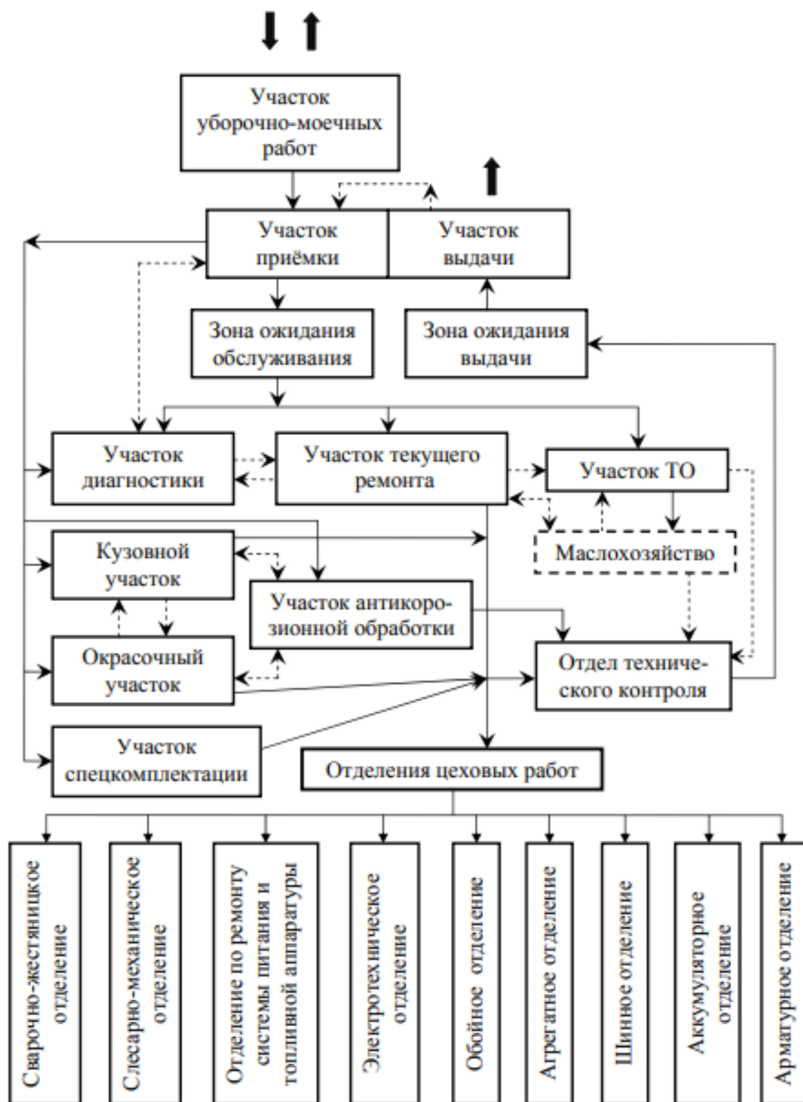
Схема технологического процесса текущего ремонта на СТО
