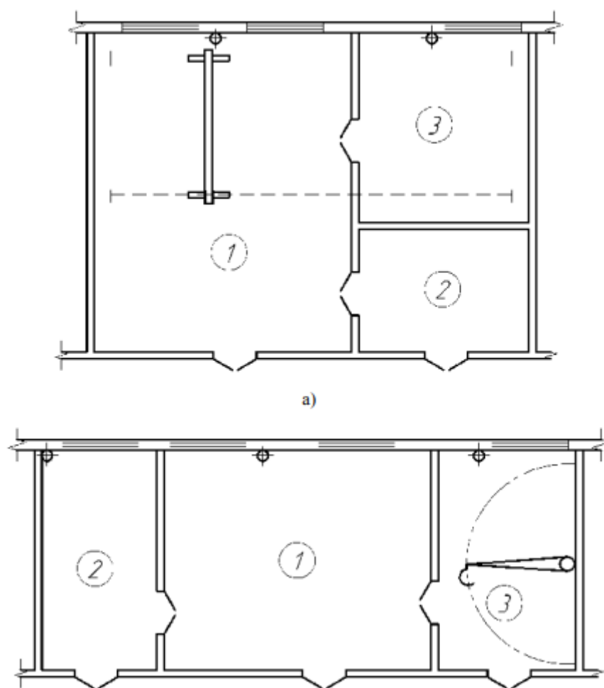
Рис. 8.16. Примеры планировочного решения агрегатного отделения Экспликация помещений: 1 – участок ремонта узлов и агрегатов, 2 – помещение для мойки агрегатов в сборе, а также для мойки и очистки узлов и деталей, 3 – помещение для обкатки отремонтированных агрегатов
