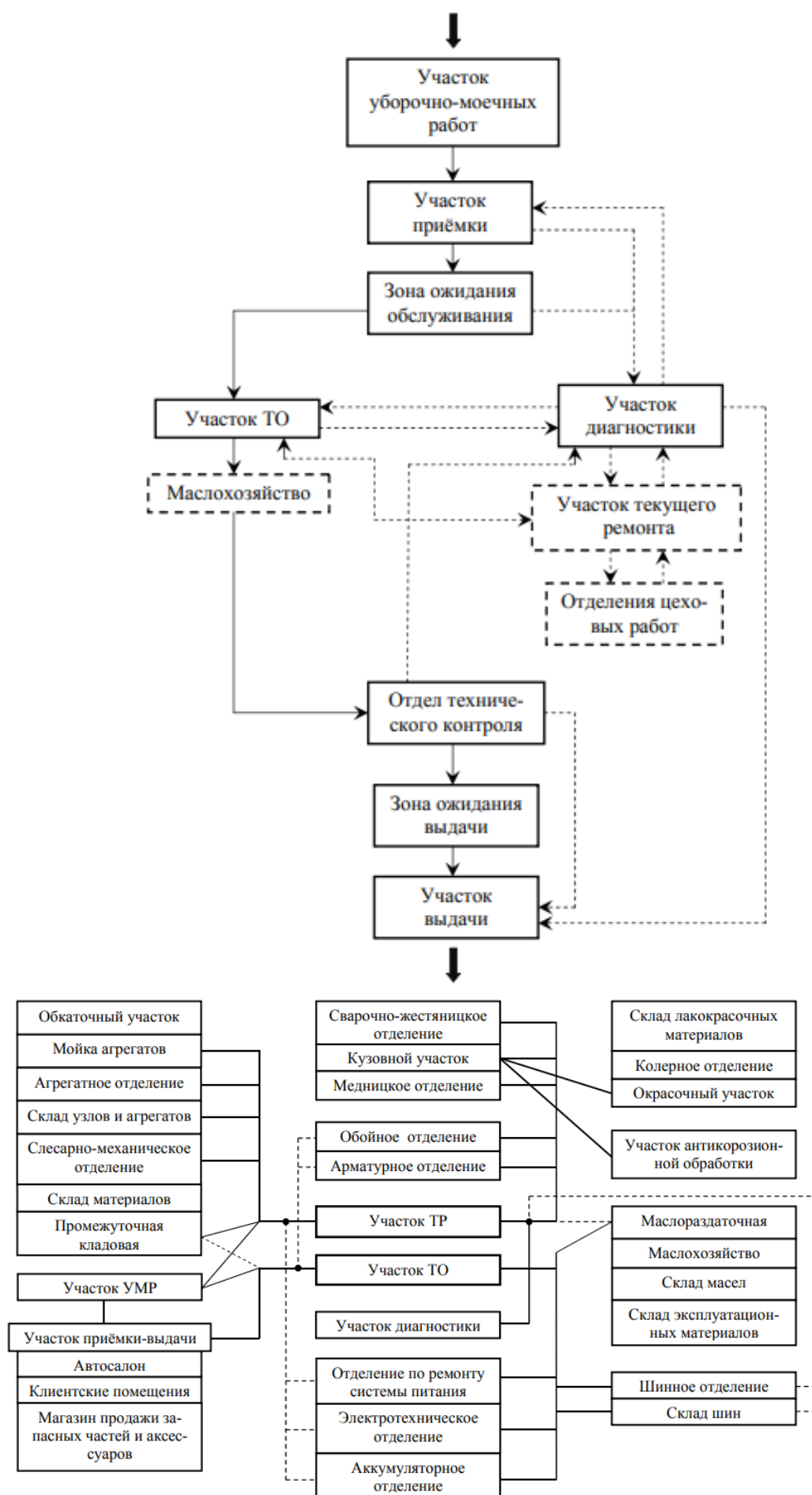
Технологические связи подразделениями сервисных предприятий
