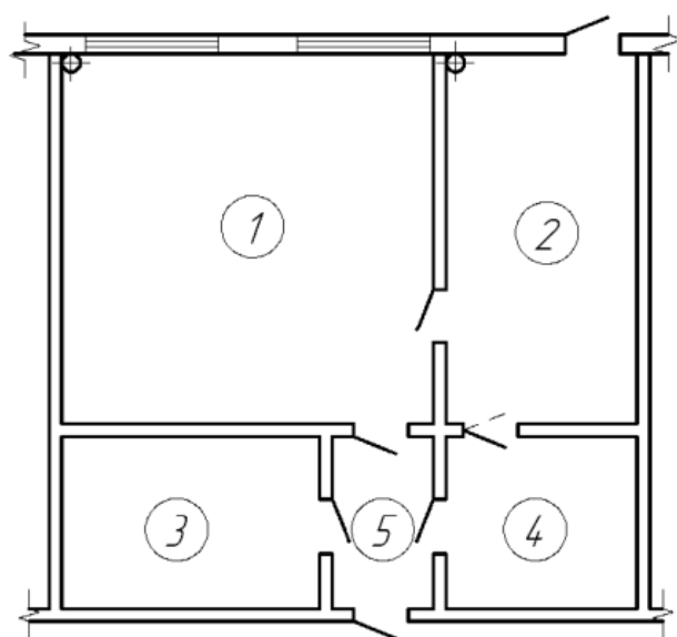
Рис. 8.17. Пример планировочного решения аккумуляторного отделения крупных СТО Экспликация помещений: 1 – участок по ремонту АКБ, 2 – зарядное помещение, 3 – помещение для хранения кислоты, 4 – аппаратная, 5 – тамбур.
