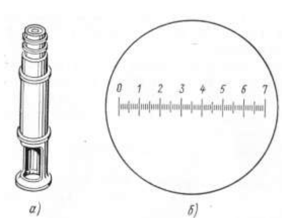
Рисунок 3 – Лупа для измерения отпечатков: а—внешний вид; б—шкала лупы
