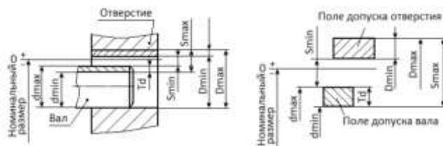
Рисунок 1 –Соединение деталей по посадке с гарантированным зазором
