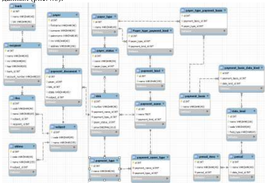
Рис.4.8. Физическая модель базы данных
