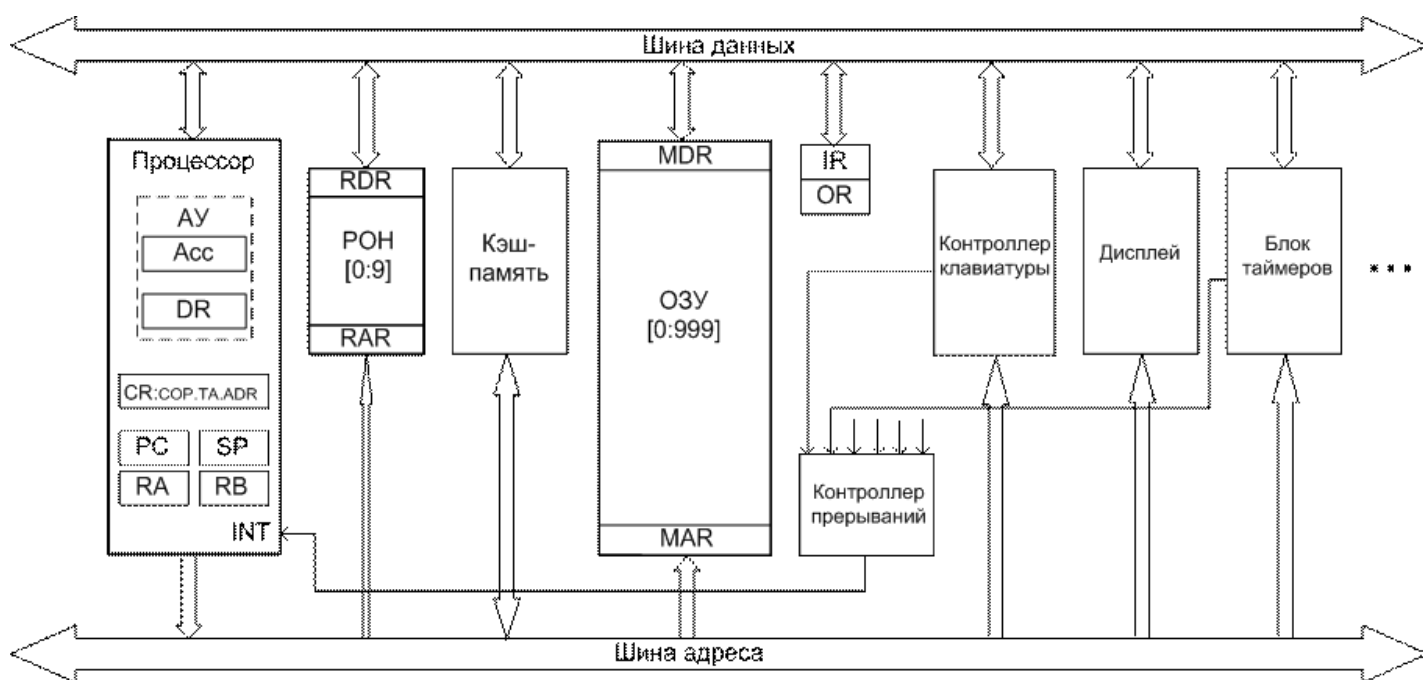
Рис.1 Общая структура учебной ЭВМ.
