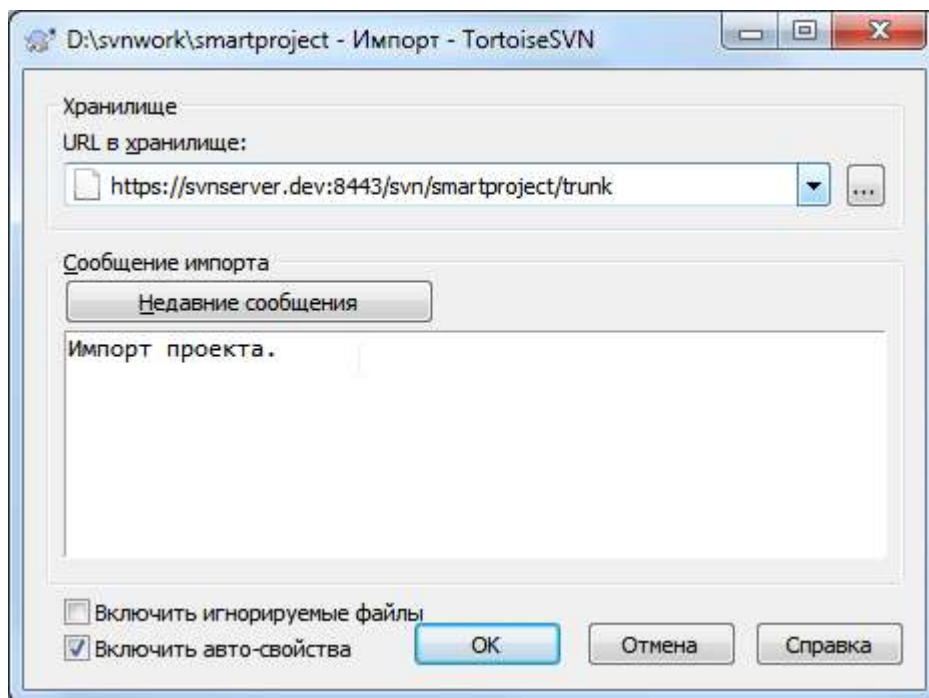
Рис. 2. Диалог импорта
