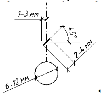
Рисунок 1 - Правила оформления координационных осей
