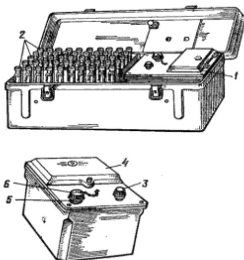
1 – зарядное устройство ЗД-5; 2 – индивидуальные дозиметры ДКП-50-А; 3 – ручка потенциометра; 4 – крышка отсека питания; 5 – зарядное гнездо; 6 – колпачок Рис. 2 – Комплект индивидуальных дозиметров ДП-22В
