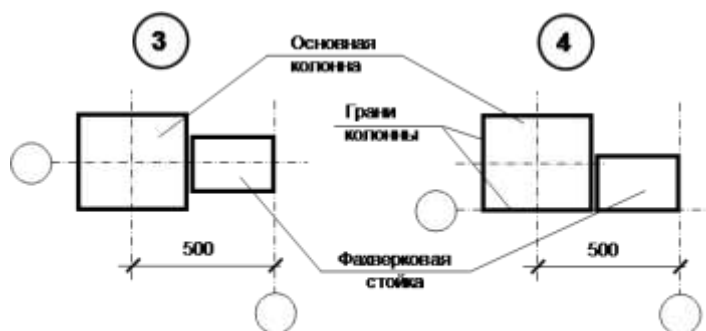
Рис. 3.5. Привязка «500»
