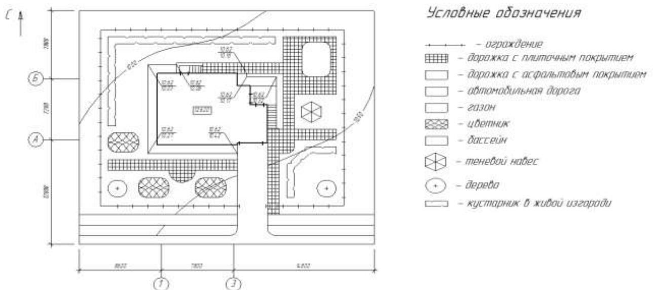
Рисунок 8.1 Генплан М 1:500
