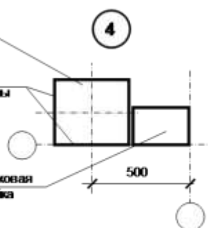
Рис. 3.6. Привязка «500»
