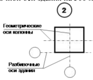
Рис. 3.4. Нулевая привязка
