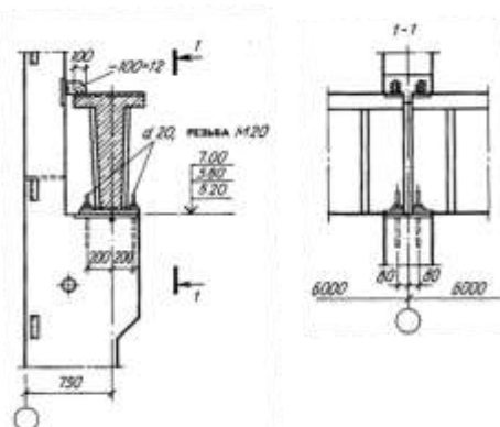
Рис. 4.5. Узел опоры подкрановой балки
