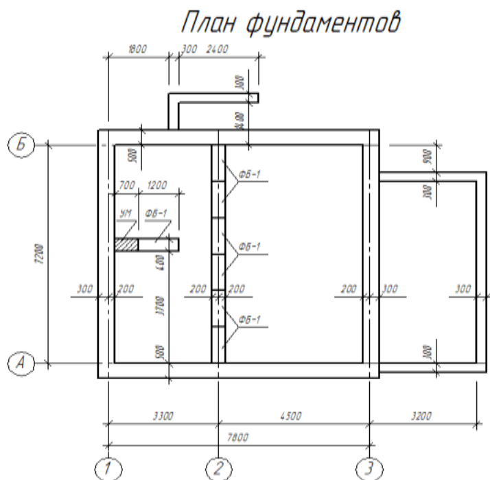
Рисунок 2.1 Пример выполнения плана фундаментов
