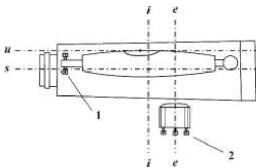
Рисунок 18. Оси и исправительные винты нивелира: ss – визирная ось зрительной трубы; ii – ось вращения прибора; uu – ось цилиндрического уровня; ee – ось круглого уровня; 1 – исправительные винты цилиндрического уровня; 2 – исправительные винты круглого уровня.
