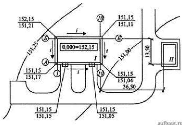
Рисунок 4. Пример выполнения вертикальной и горизонтальной привязок в учебной практической работе: I - проектируемое здание; II - существующее здание; i - направление стока поверхностных вод; A, Б, 1, 10 - обозначения осей
