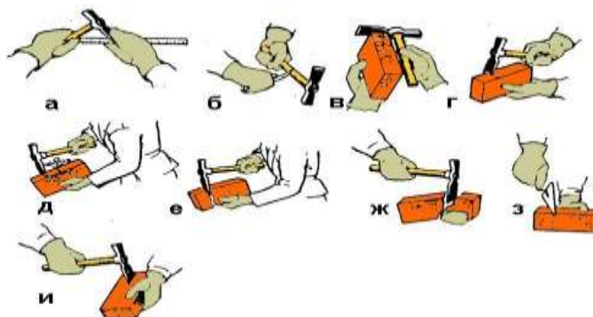
Рисунок 1. Приемы рубки кирпича:
