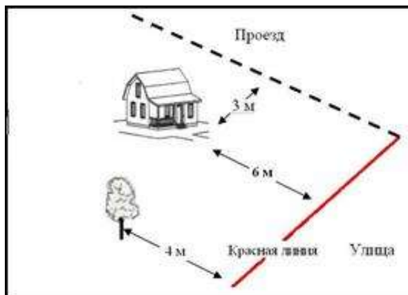
Рисунок 17.1 – Нормы и требования при планировке участка
