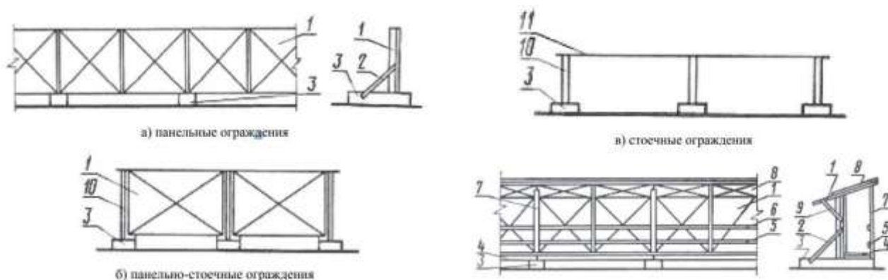
Рисунок 20.1 - Схемы ограждений
