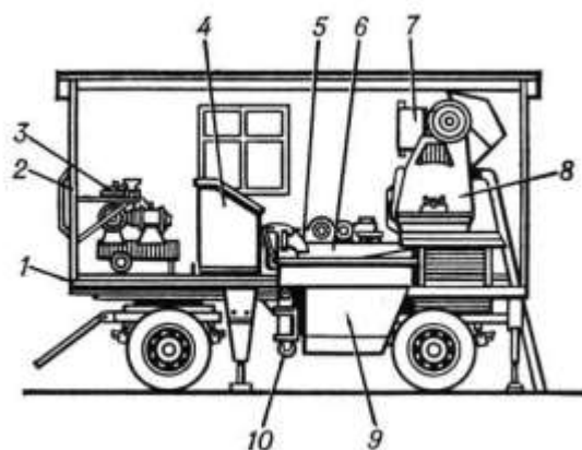
Рисунок 4. Передвижная штукатурная станция: 1 — площадка автоприцепа; 2 — патрубков; 3 — компрессор; 4 — пульт управления; 5, 10 — растворонасосы; 6 — виброрито; 7 — дозировочный бак; 8 — растворосмеситель; 9 — промежуточный бункер.
