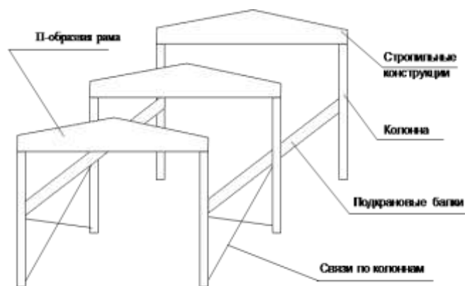
Рис. 3.1. Каркас здания
