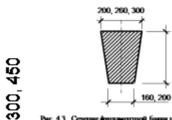
Рис. 4.3. Сечение фундаментной базы при шаге колонн 6 м
