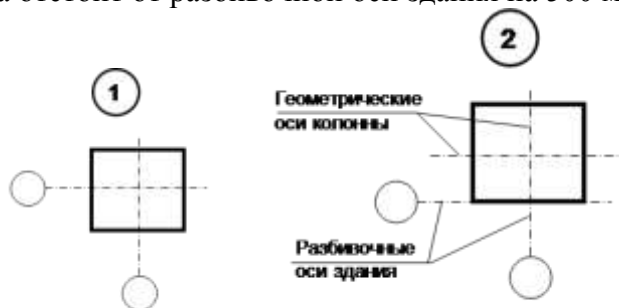
Рис. 3.4. Нулевая привязка
