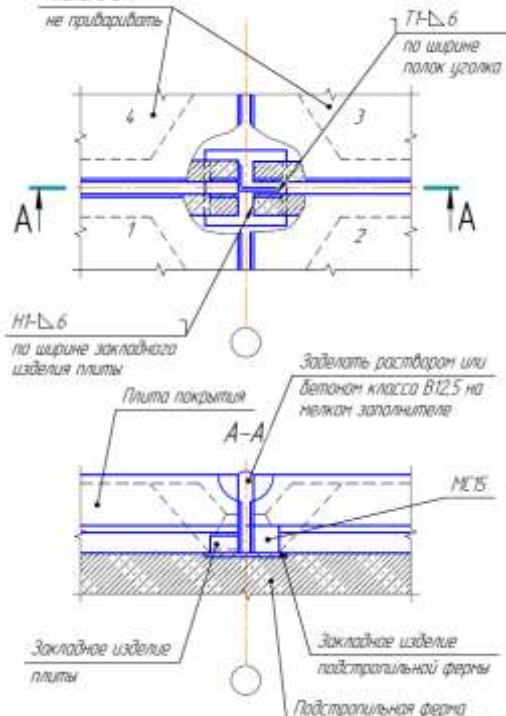
Крепление плит покрытия к подстропильной ферме в пролете Плиты 3 и 4 не приваривать
