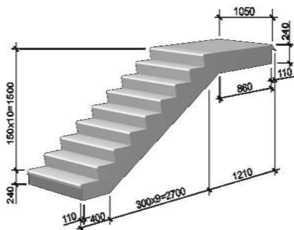
Рис. 9.20. Лестничные марши железобетонные совмещенные с лестничными площадками
