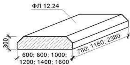
Фундаментная подушка
