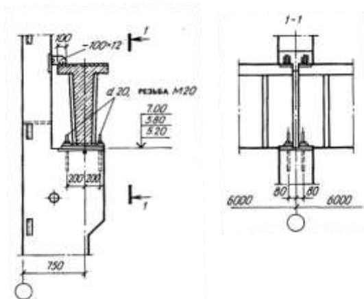
Рис. 4.5. Узел опоры подкрановой балки
