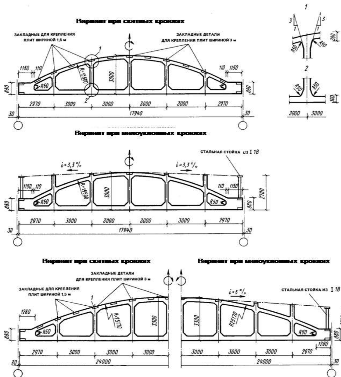
Рис. 4.8. Стропильные фермы (пролеты 18 и 24 м)
