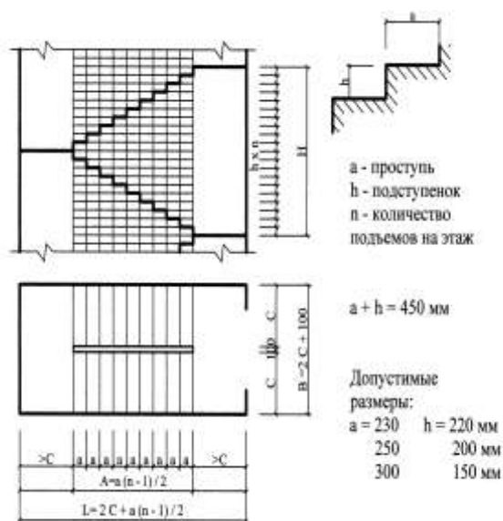
Рис. 3.3. Расчет лестничной клетки
