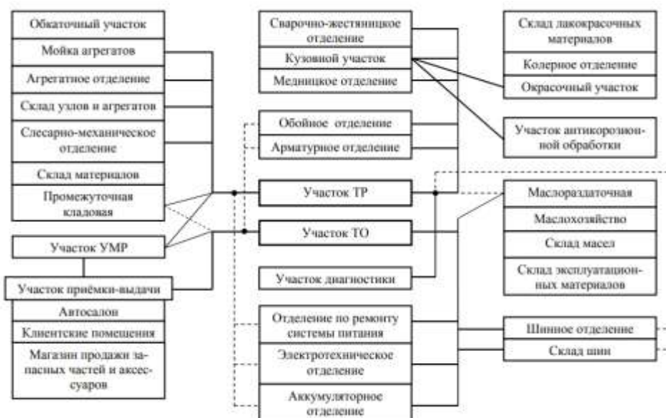
Технологические связи подразделениями сервисных предприятий
