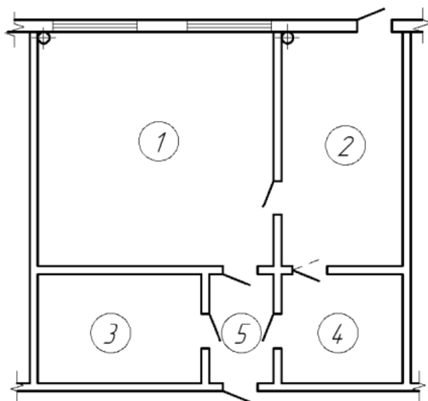
Рис. 8.17. Пример планировочного решения аккумуляторного отделения крупных СТО
