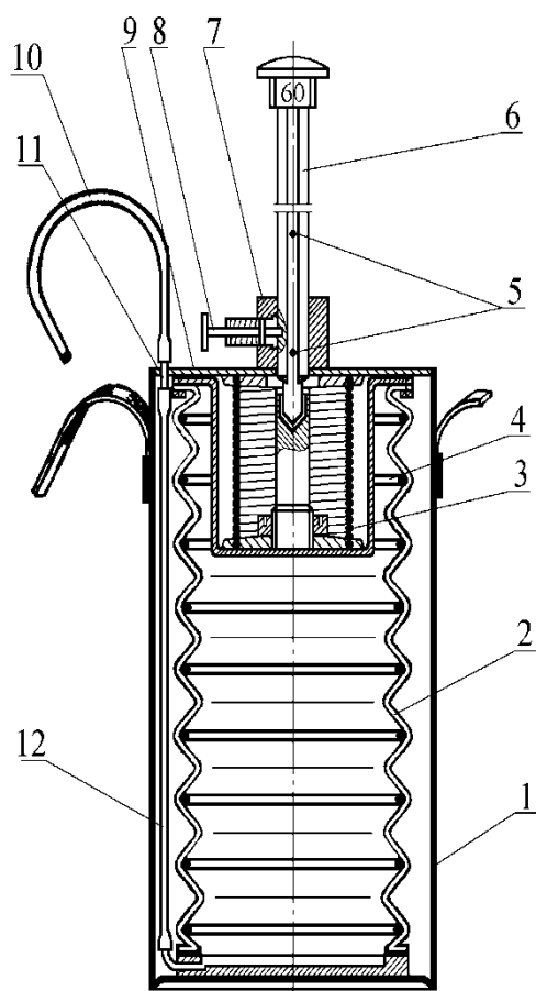
Рис. 1. Устройство газоанализатора
