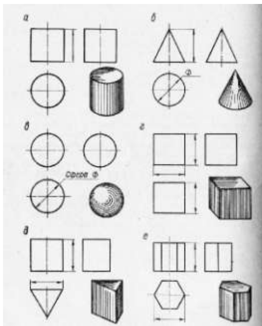
Рис.10 Проекция геометрических тел призмы
