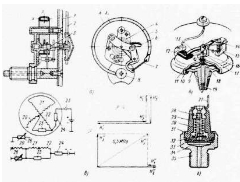
Рисунок 2. Указатель давления: а) механизм указателя с трубчатой пружиной; б) Реостатный датчик магнитоэлектрического приёмника; в) Электрическая схема магнитоэлектрического приёмника и диаграмма векторов напряжённости; г) Датчик ММ - 124Б аварийного давления.
