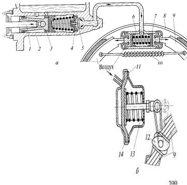
Рис.17.1 Схема тормозного механизма с приводом:
