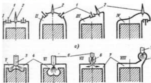
Рис. 1. Формы камер сгорания: а — карбюраторных двигателей; б — дизелей; I — цилиндрическая; II — полусферическая; III — клиновидная; IV — смещенная (Г-образная); V и VI — неразделенные; VII и VIII — разделенные; 1 — клапан; 2 — свеча зажигания; 3 — насос-форсунка; 4 — камера сгорания; 5 — форсунка; 6 — предкамера; 7 — основная камера; 8 — вихревая камера
