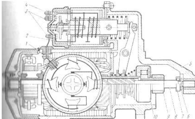
Рис 78 Стартер СТ 230
