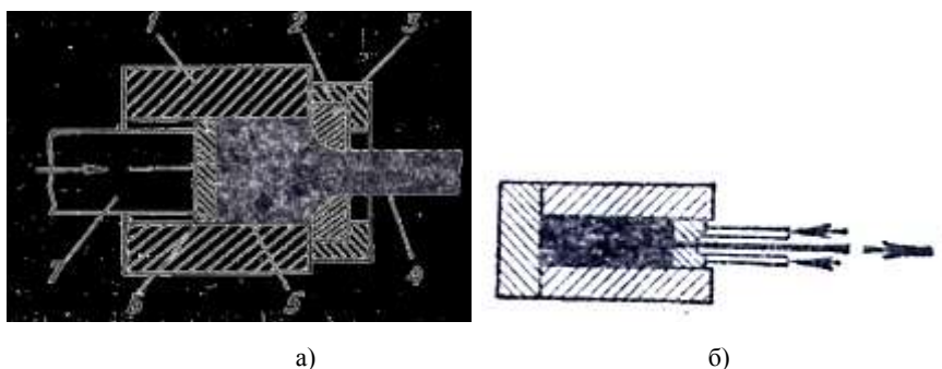
Рис.3 . Схема процесса прессования:
