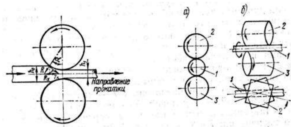
Рис.8. Схема прокатки:
