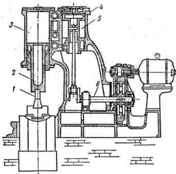
Рис. 5 Ковочный пневматический молот: 1-боек; 2-шток; 3-рабочий цилиндр; 4-поршень; 5-компрессорный цилиндр; 6-кривошип
