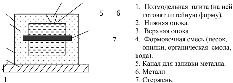
Рис. 1. Литейная форма
