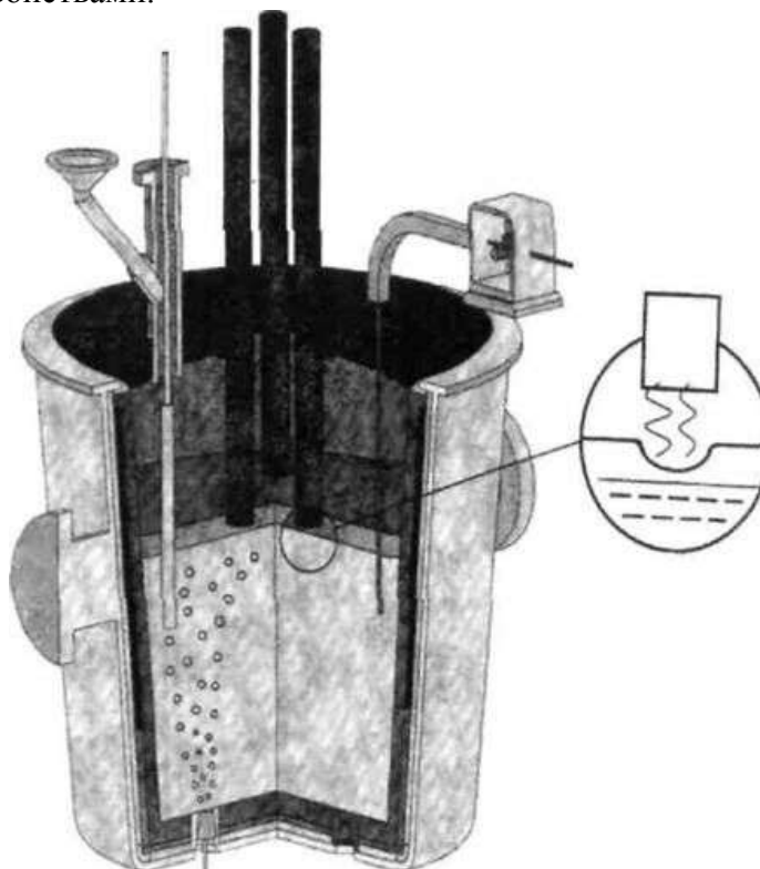
Рисунок 1 - Агрегат ковш-печь (АКП).
