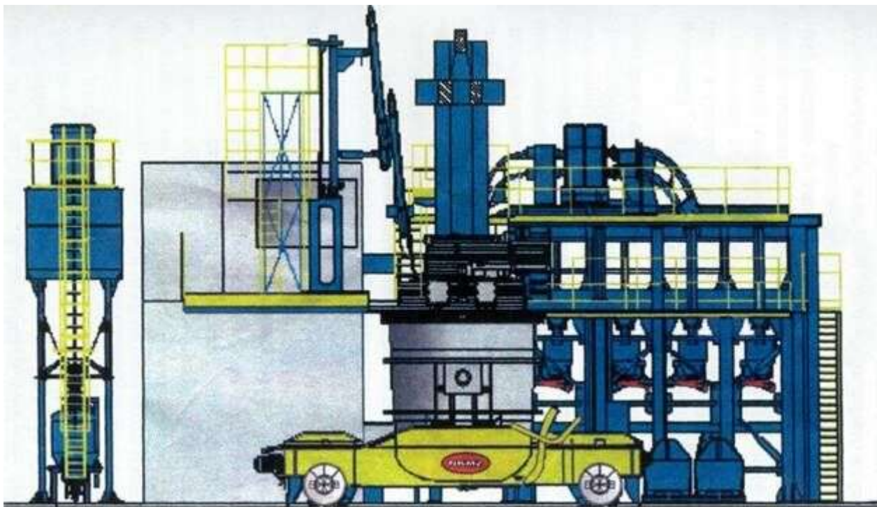
Рисунок 3 - Расположение оборудования агрегата ковш-печь поперек цеха
