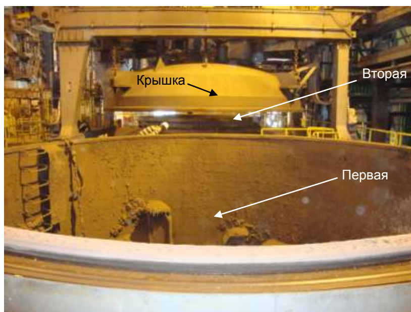
Рисунок 2 - Двухкамерный вакууматор фирмы «Danieli» в компании «ММК-Metalurji»
