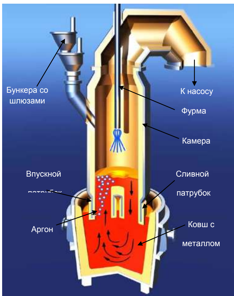
Рисунок 3 - Циркуляционный вакууматор типа RH
