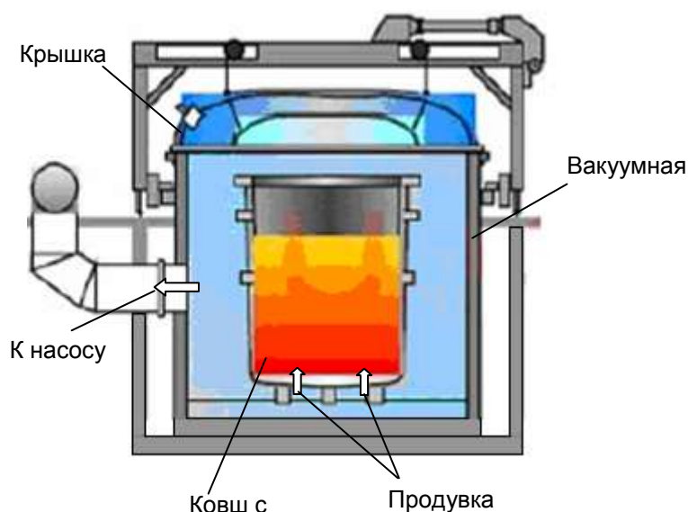
Рисунок 1 - Схема вакууматора камерного типа
