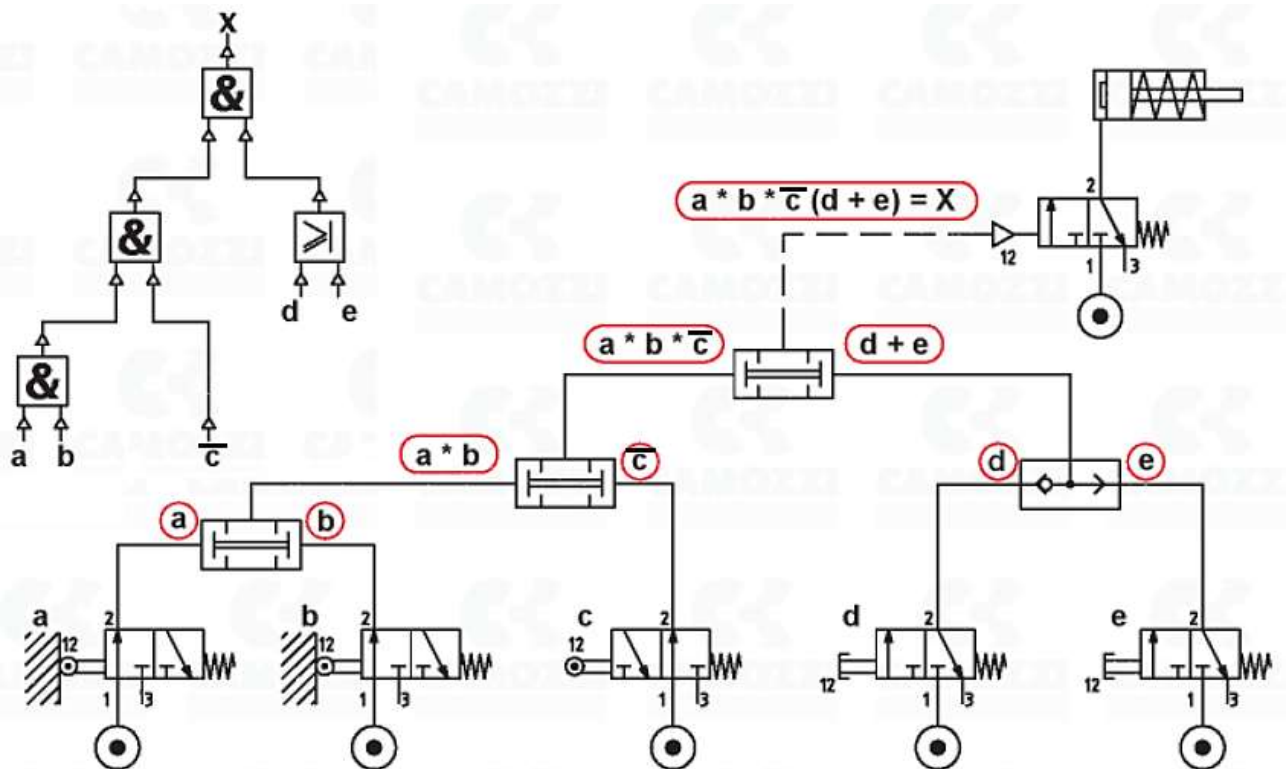
Рисунок 15 – Схема пневматическая принципиальная
