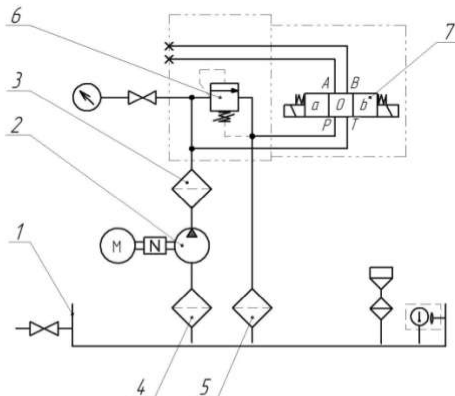
1. Бак 2. Насос 3.Фильтр напорный 4.Фильтр всасывающий 5.Фильтр сливной 6.Предохранительный клапан 7.Гидрораспределитель
