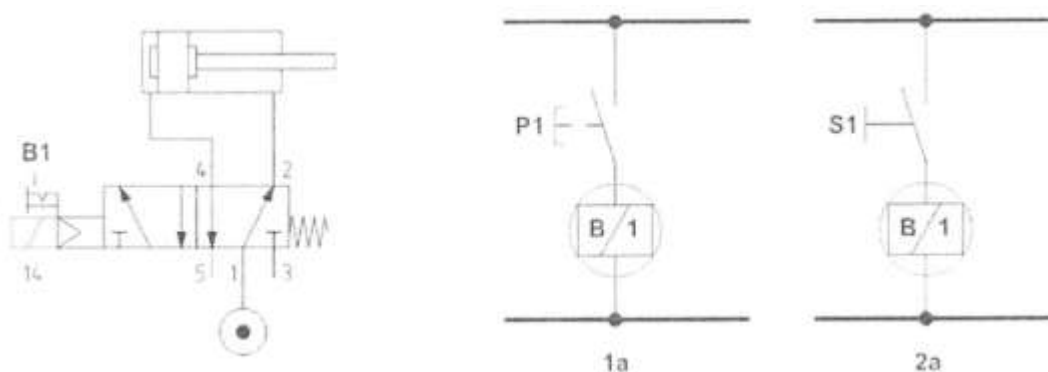
Рисунок 35 Электропневматическая схема
