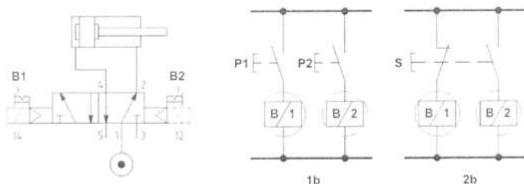
Рисунок 36 Электропневматическая схема
