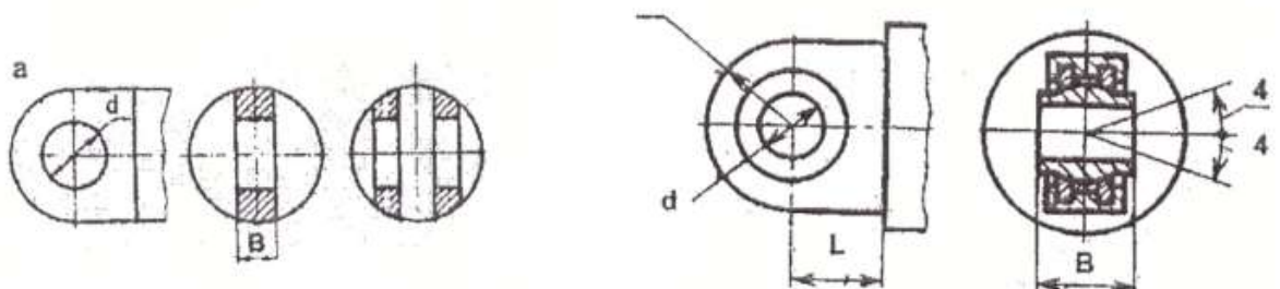
Рисунок 19.1 – Конструкция проушины
