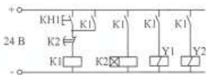
Рисунок 24.2 Схема электрическая
