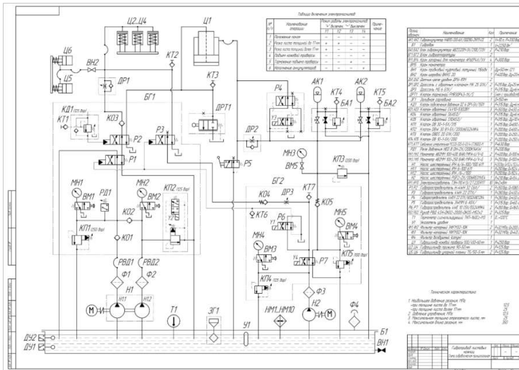
Рисунок 10.2– Гидросхема листовых ножниц
