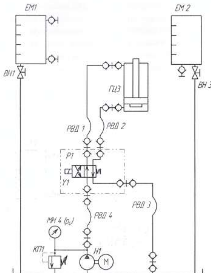
Рисунок 20.1 Схема гидравлическая
