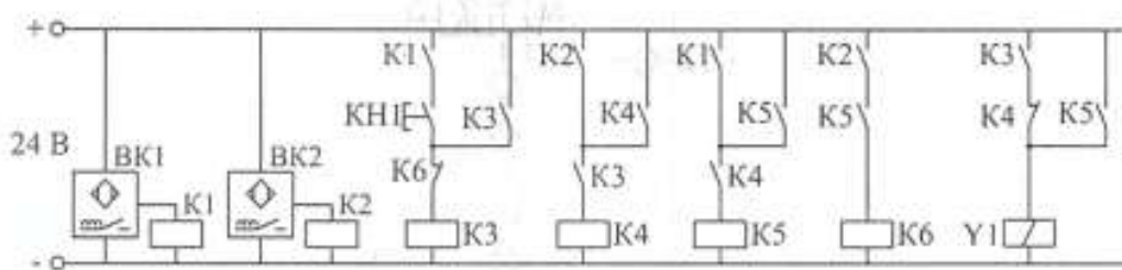
Рисунок 25.2 Схема электрическая
