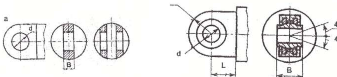
Рисунок 28.1 – Конструкция проушины
