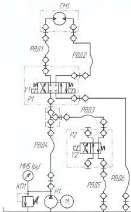
Рисунок 24.1 –Схема гидравлическая
