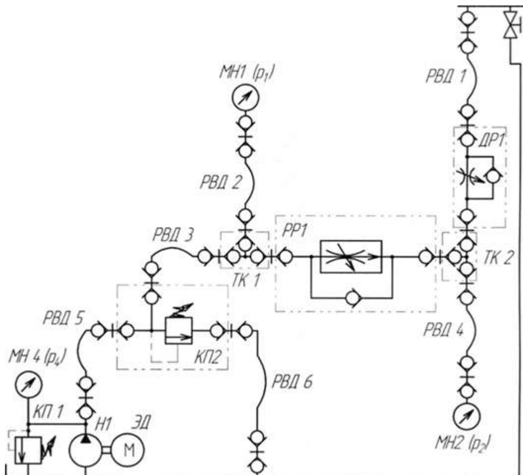
Рисунок 10 – гидравлическая схема
