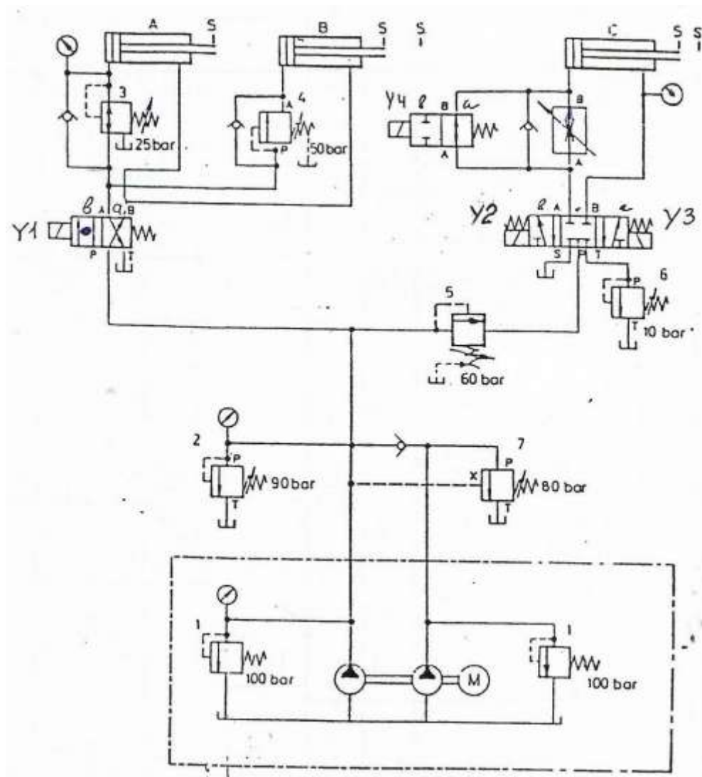
Рисунок 9.1 – Гидросхема гибочного станка
