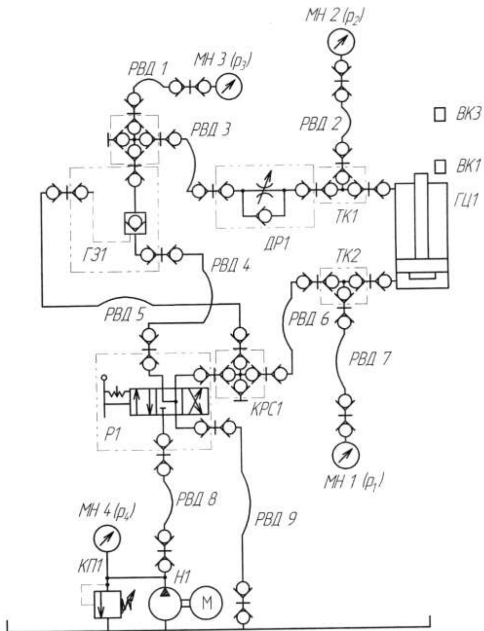
Рисунок 14.1 – схема гидравлическая
