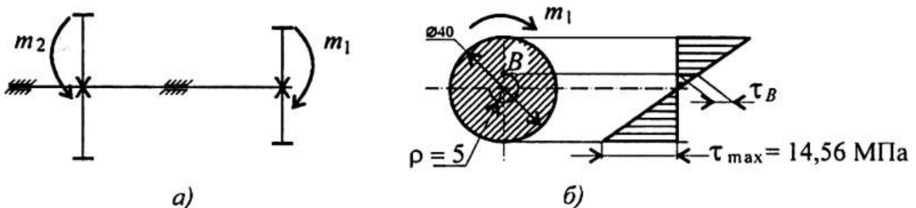
Рисунок 1 – Схема вала
