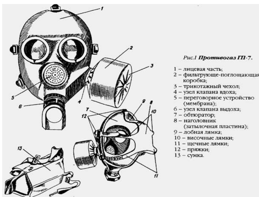
Рисунок 1 Противогаз ГП-7.
