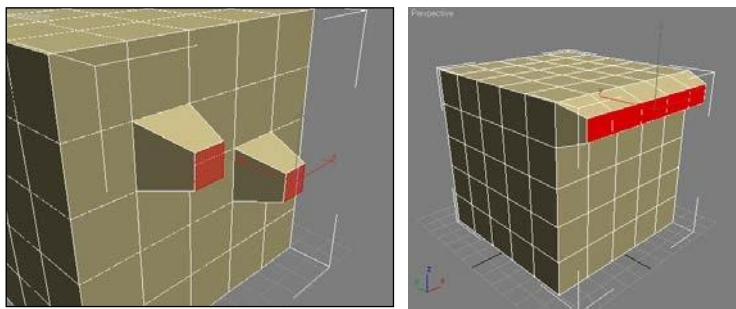
Рис. 9.14. Инструмент Bevel
