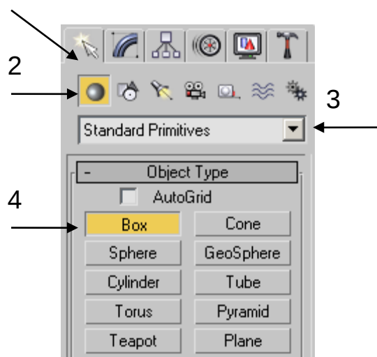
Рис. 3.1. Командная панель
