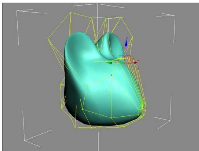
Рис. 1.6. Пример NURBS-поверхности
