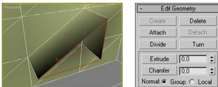
Рис. 9.11. Функция Extrude
