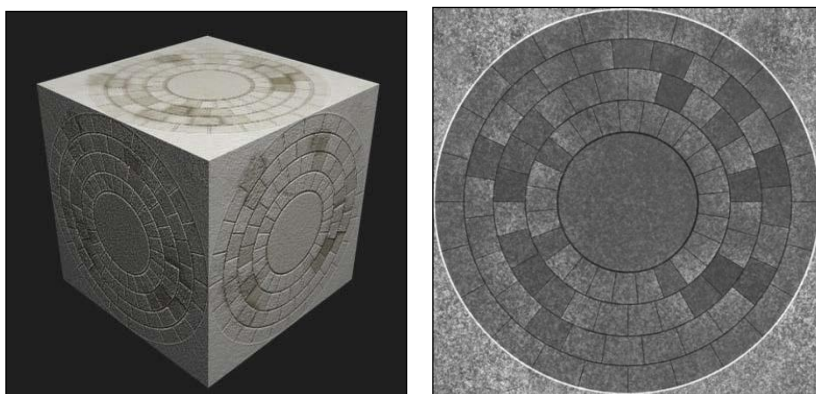
Рис. 1.8. Получение рельефности
