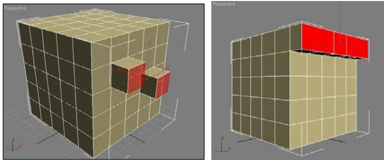
Рис. 9.13. Выдавливание полигонов
