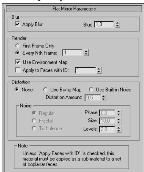
Рис. 10.24. Настройки карты Flat Mirror
