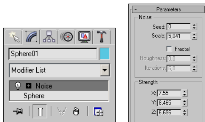
Рис. 10.31. Модификатор Noise
