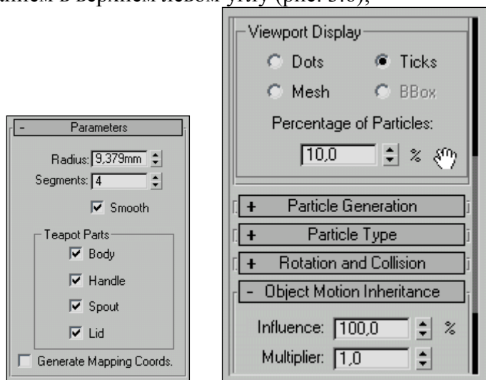
Рис. 3.6. Подгруппа параметров
