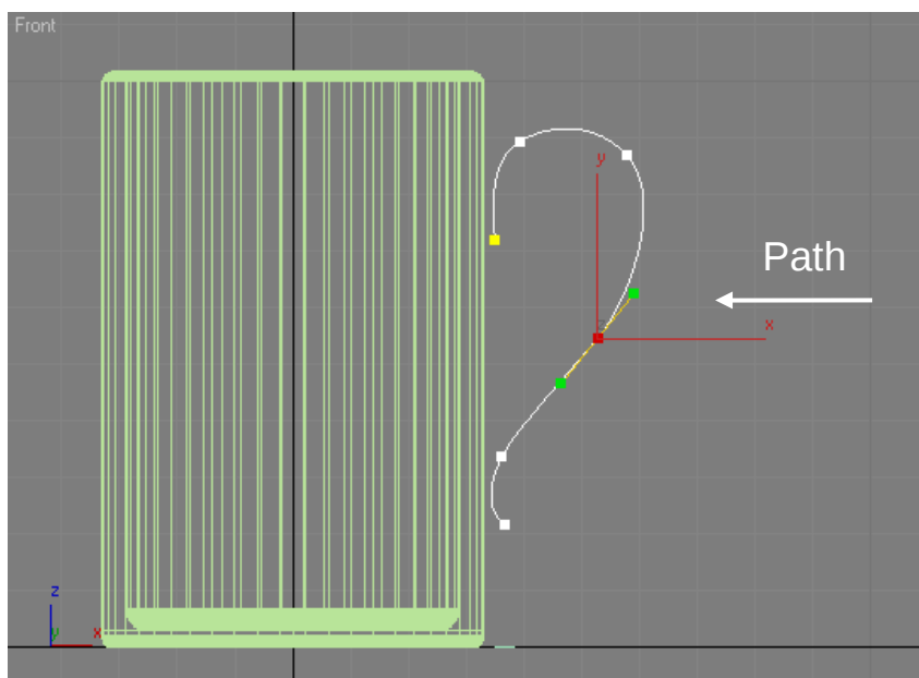
Рис. 8.1. Форма ручки
