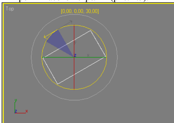
Рис. 4.5. Поворот объекта
