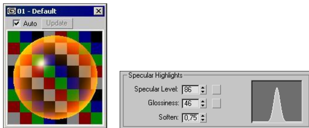
Рис. 10.30. Задание блика
