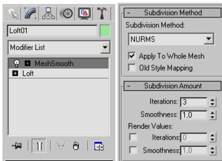
Рис. 8.11. Стек модификаторов
