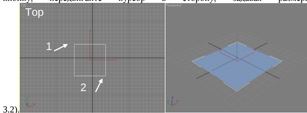
Рис. 3.2. Основание параллелепипеда
