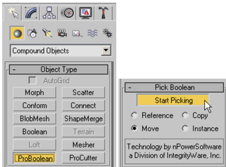
Рис. 8.18. Панель команд
