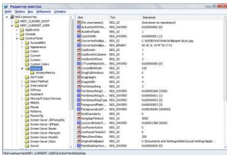
Рисунок 2. Ключ реестра отвечающий за настройки рабочего стола.
