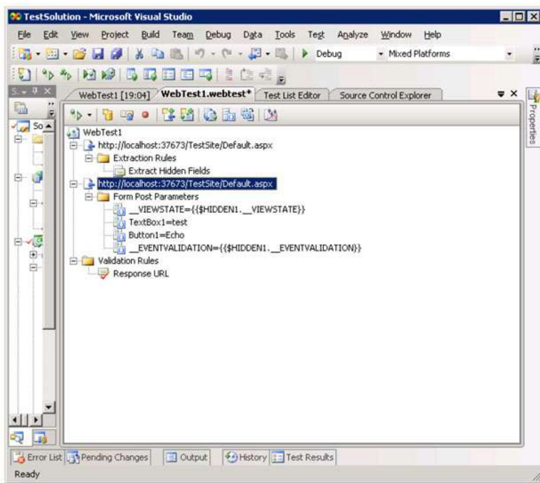
Рисунок 10 – Редактор Web-теста
