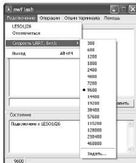
Рисунок 53 – Настройка скорости UART
