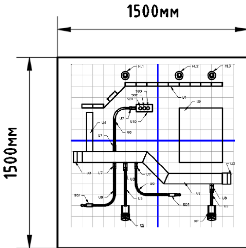
Рисунок 1 – Схема расположения электрооборудования
