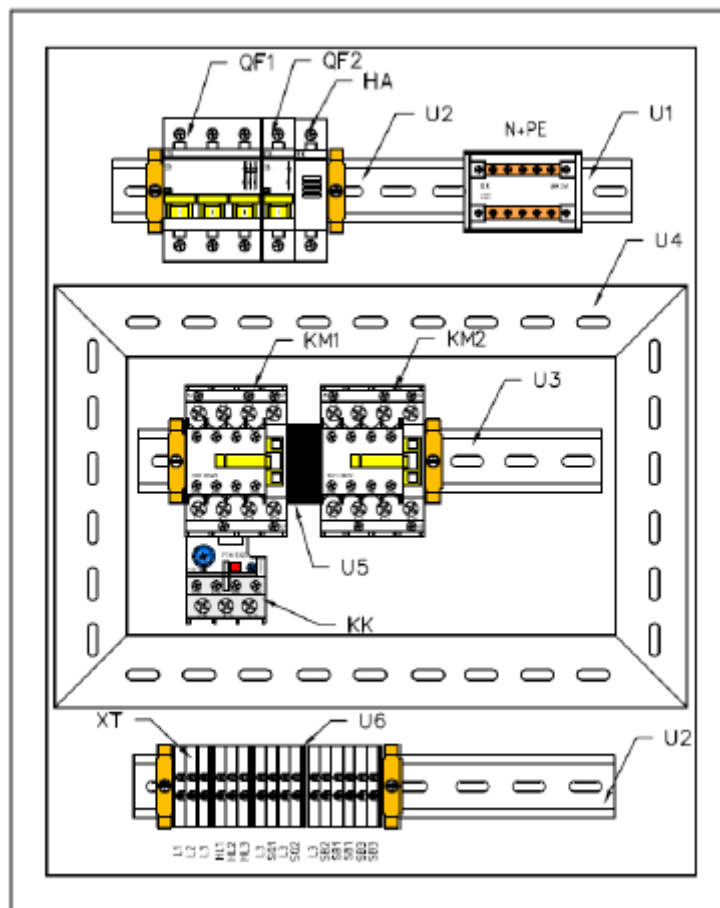
Рисунок 2 – Схема расположения электрооборудования в ЩУ
