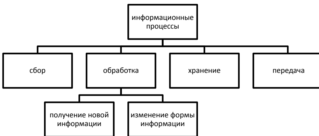
Рисунок 3 – Информационные процессы
