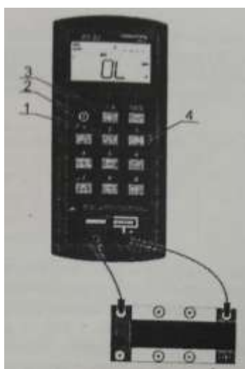
Рис. 1. Соединение измерителя RLC и минимодуля "Диэлектрическая проницаемость": 1 – кнопка выбора режима измерения основного параметра, 2 – кнопка включения прибора, 3 – кнопка выбора частоты тест-сигнала, 4 – кнопка выбора режима измерения дополнительного параметра
