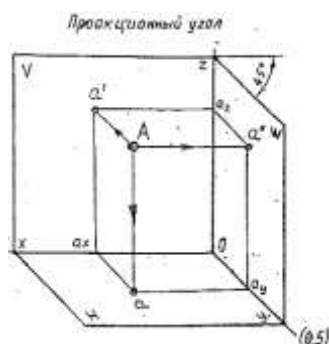
Рис.4 Проекция точки
