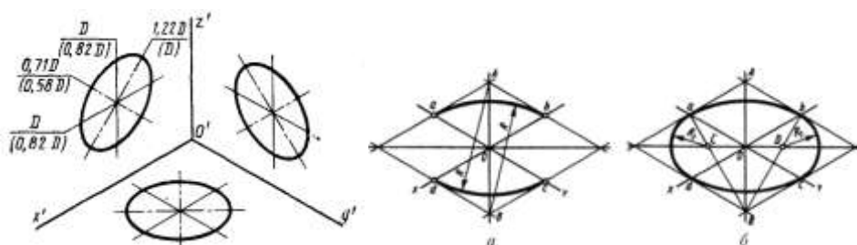
Рис.26 Аксонометрия окружности
