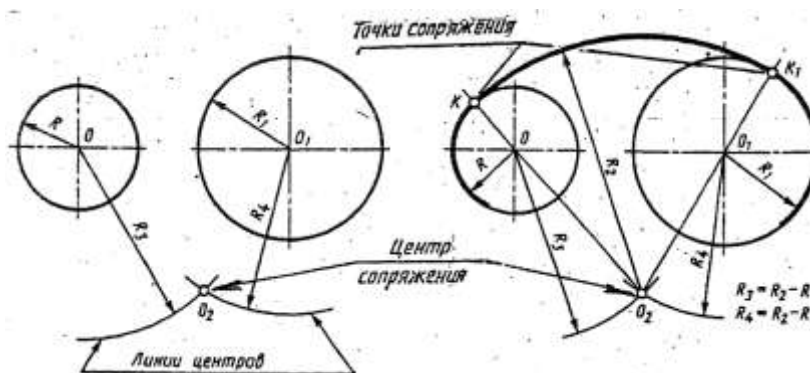
Рис.19 Внутреннее касание
