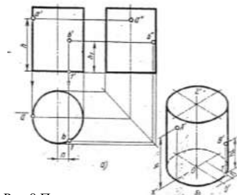
Рис.8 Проекция прямого цилиндра
