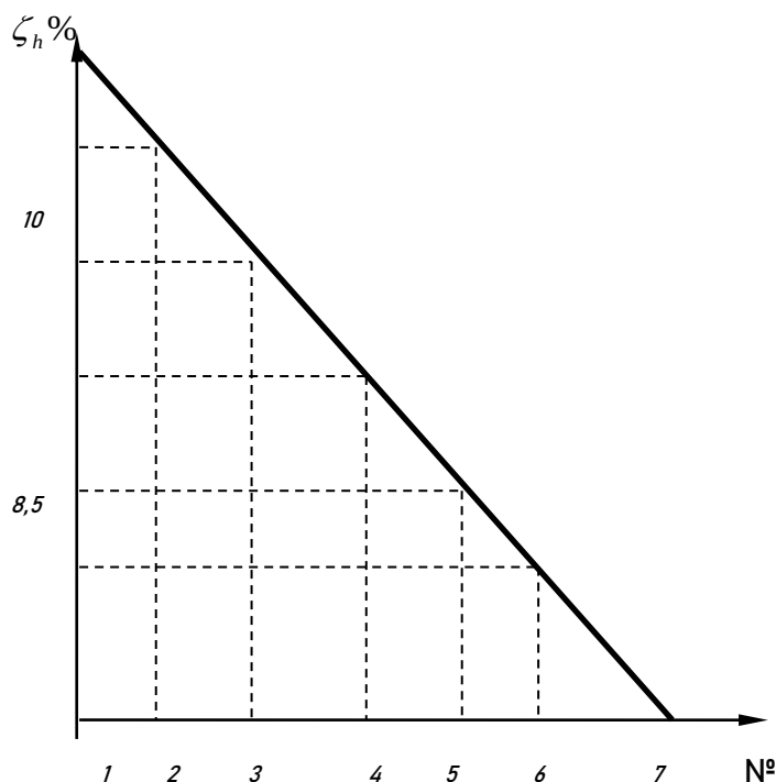
Рисунок 8 - График для значений относительной деформации по клетям чистовой группы стана
