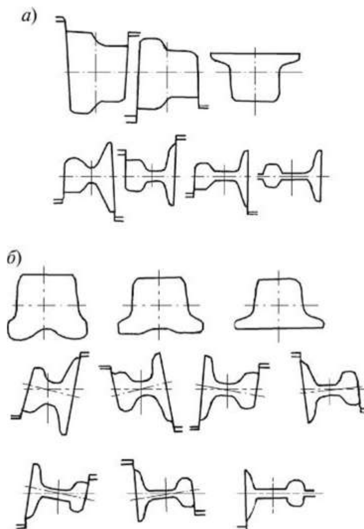
Рисунок 19 - Схемы прокатки рельсов
