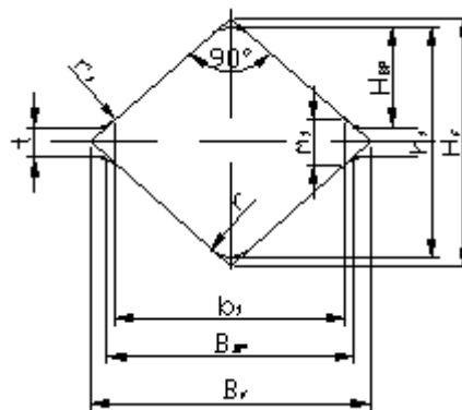
Рисунок 21 - Построение квадратного калибра
