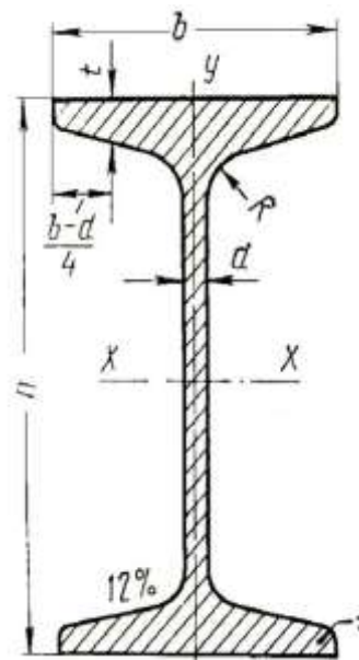
Рисунок 12 – Профиль двутавровой балки
