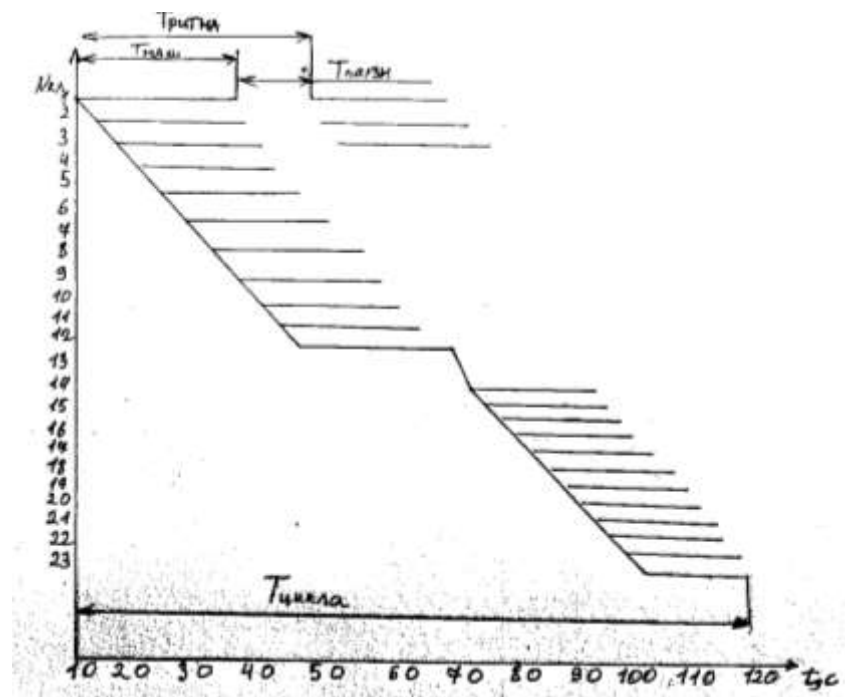
Риунок 24 - График прокатки
