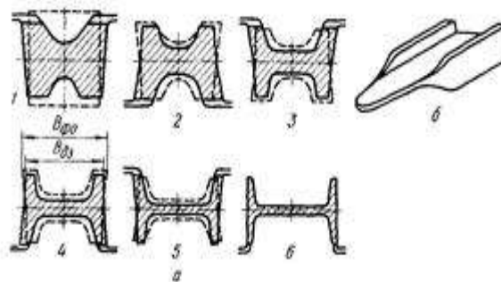
Рисунок 14 – Схемы прокатки балок малых размеров
