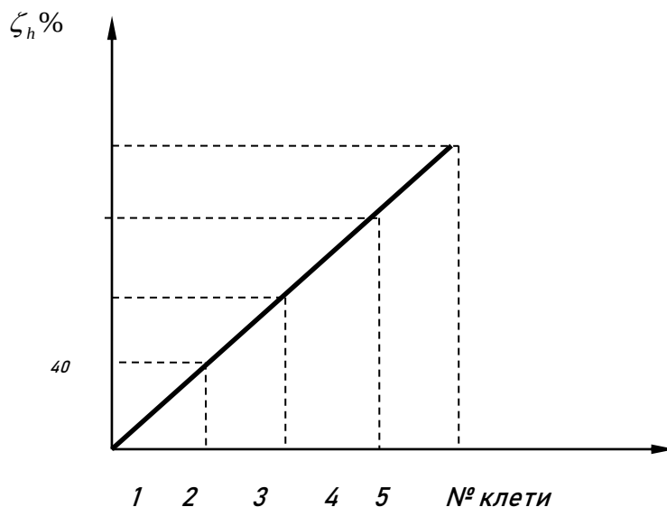
Рисунок 7 - График значений относительной деформации по проходам (клетям) при прокатке на черновой группе клетей стана
