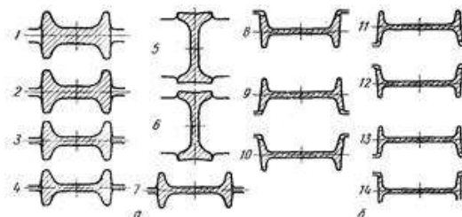
Рисунок 15 – Схемы прокатки балок крупных и средних размеров
