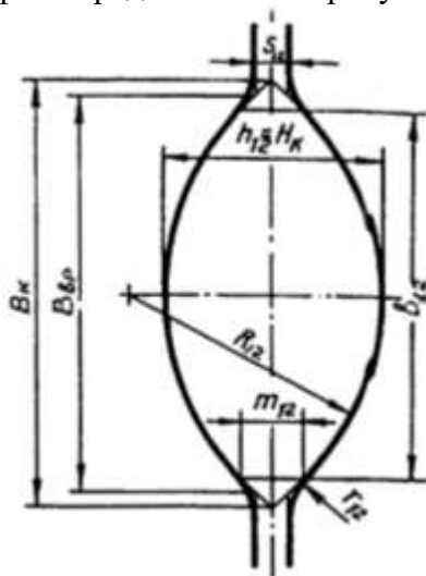
Рисунок 23 - Построение однорадиусного овального калибра.
