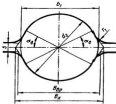
Рисунок 22 - Построение чистового круглого калибра.
