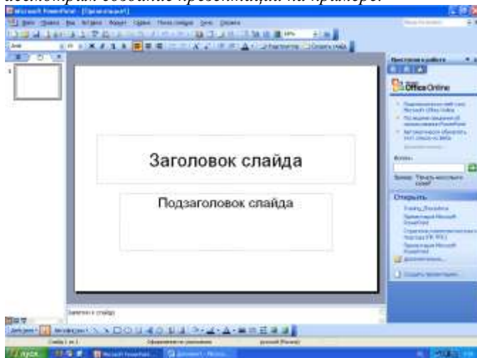
Рисунок 3.1 – Интерфейс программы
