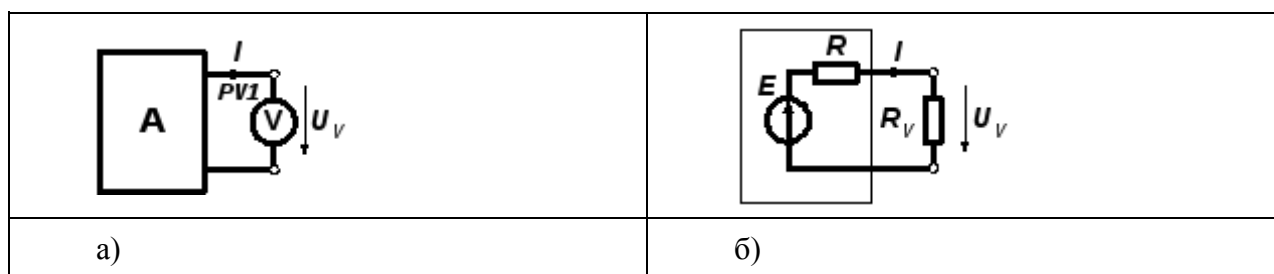
Рис. 1. Схема подключения вольтметра к исследуемой цепи (а) и эквивалентная схема измерительной цепи с вольтметром (б).
