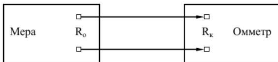
Рисунок 2 – Калибровочная схема
