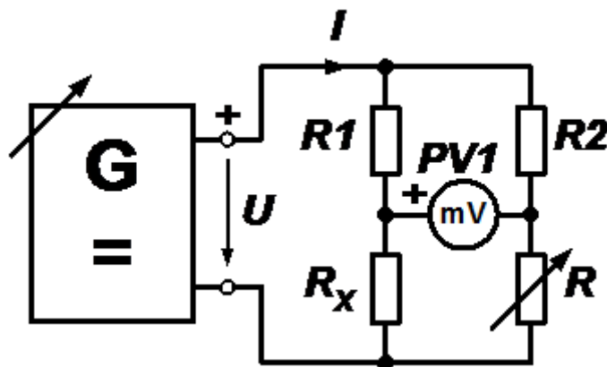
Рис. 1. Принципиальная схема измерения сопротивления с помощью моста.
