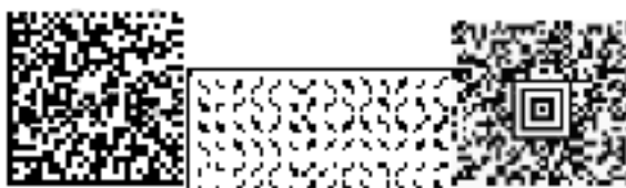
Рисунок 2 – Двухмерный штрих-код
