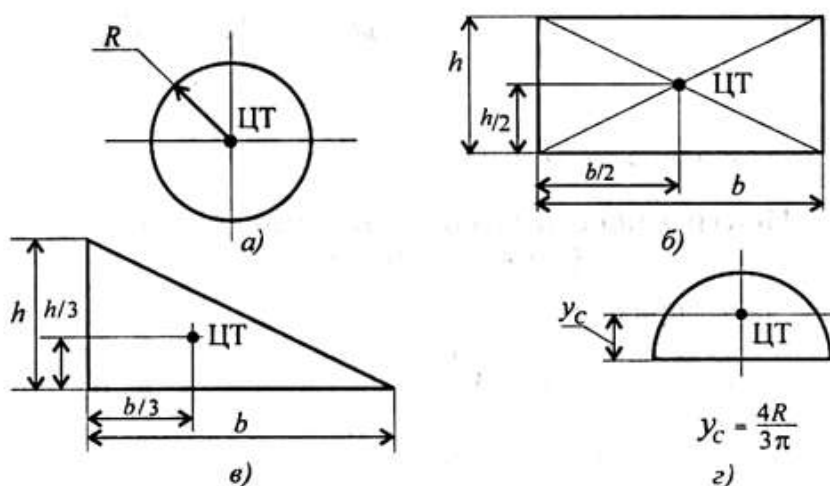
Рисунок 1 – Положения центра тяжести простых фигур:
