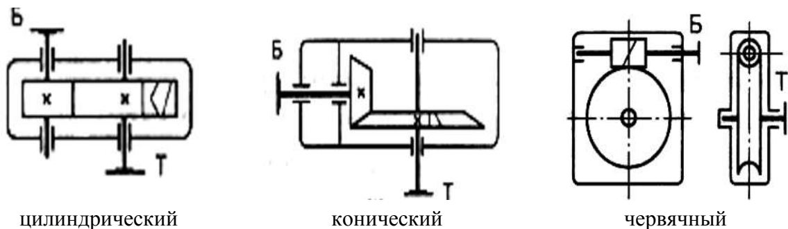
Рисунок 1 – Кинематические схемы редукторов
