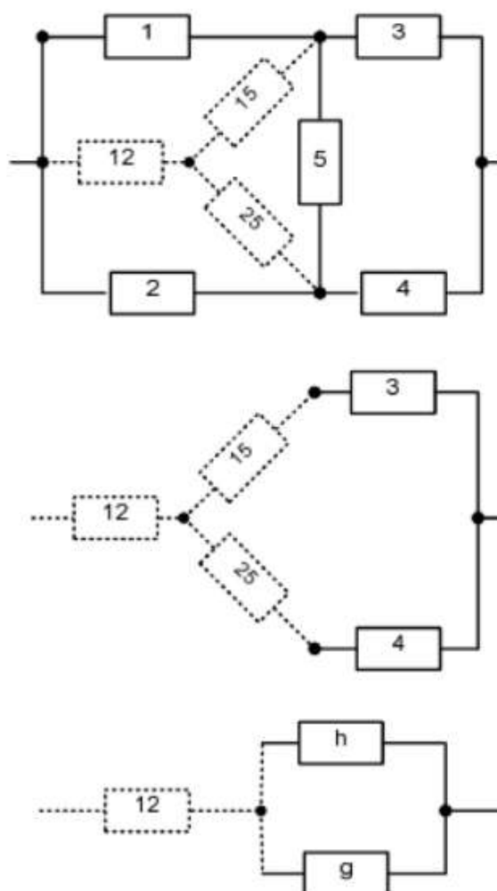
Рис. 4.4. Преобразование треугольника элементов в звезду
