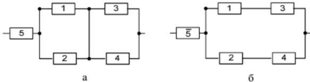
Рис. 3.2. Структурные схемы с абсолютно надёжным (а) и абсолютно не надёжным (б) базовым элементом 5
