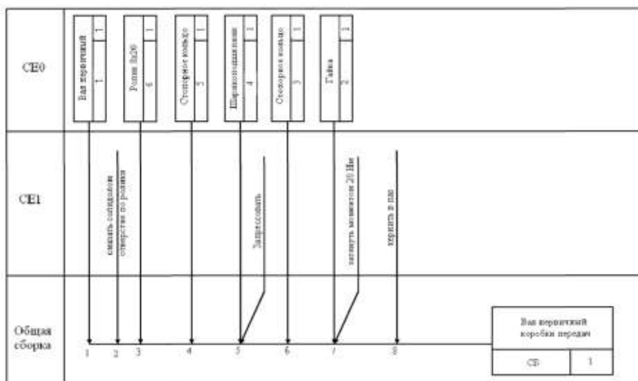
Рис. 6. Технологическая схема
