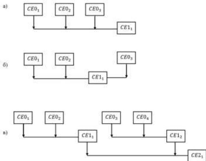
Рис 4. Схема формирования порядка сборочных
