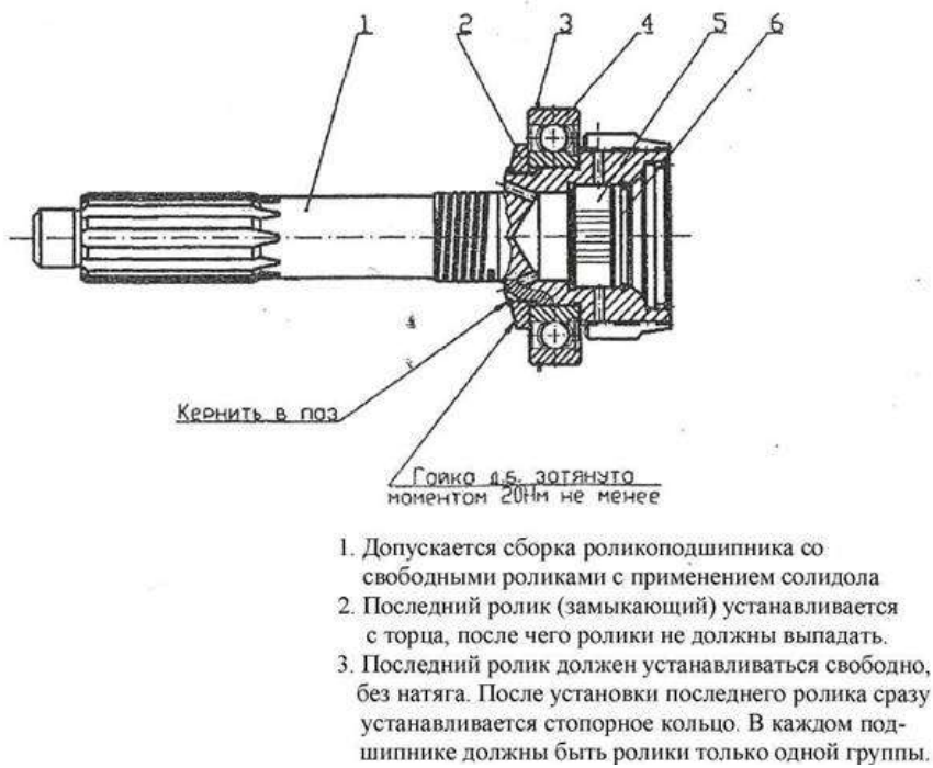
Рис 2. Первичный вал коробки передач автомобиля в сборе 1 - первичный вал; 2 - гайка; 3 - стопорное кольцо; 4 - шарикоподшипник радиальный однорядный; 5 - кольцо стопорное; 6 - ролик 8х20.
