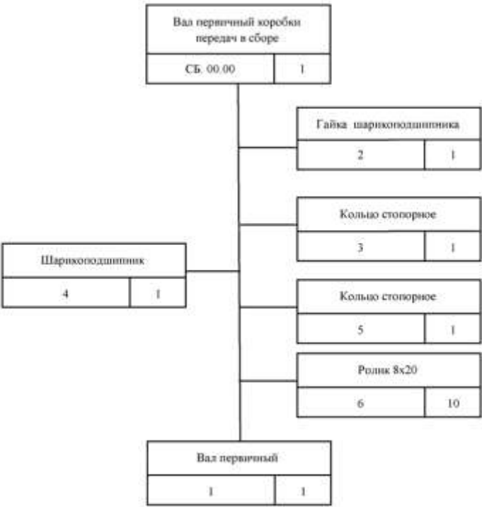
Рис.3. Технологическая схема разборки вала первичного в сборе
