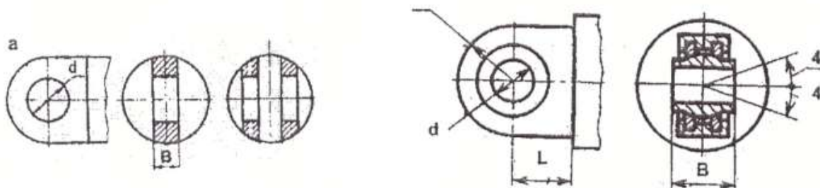
Рисунок 19.1 – Конструкция проушины
