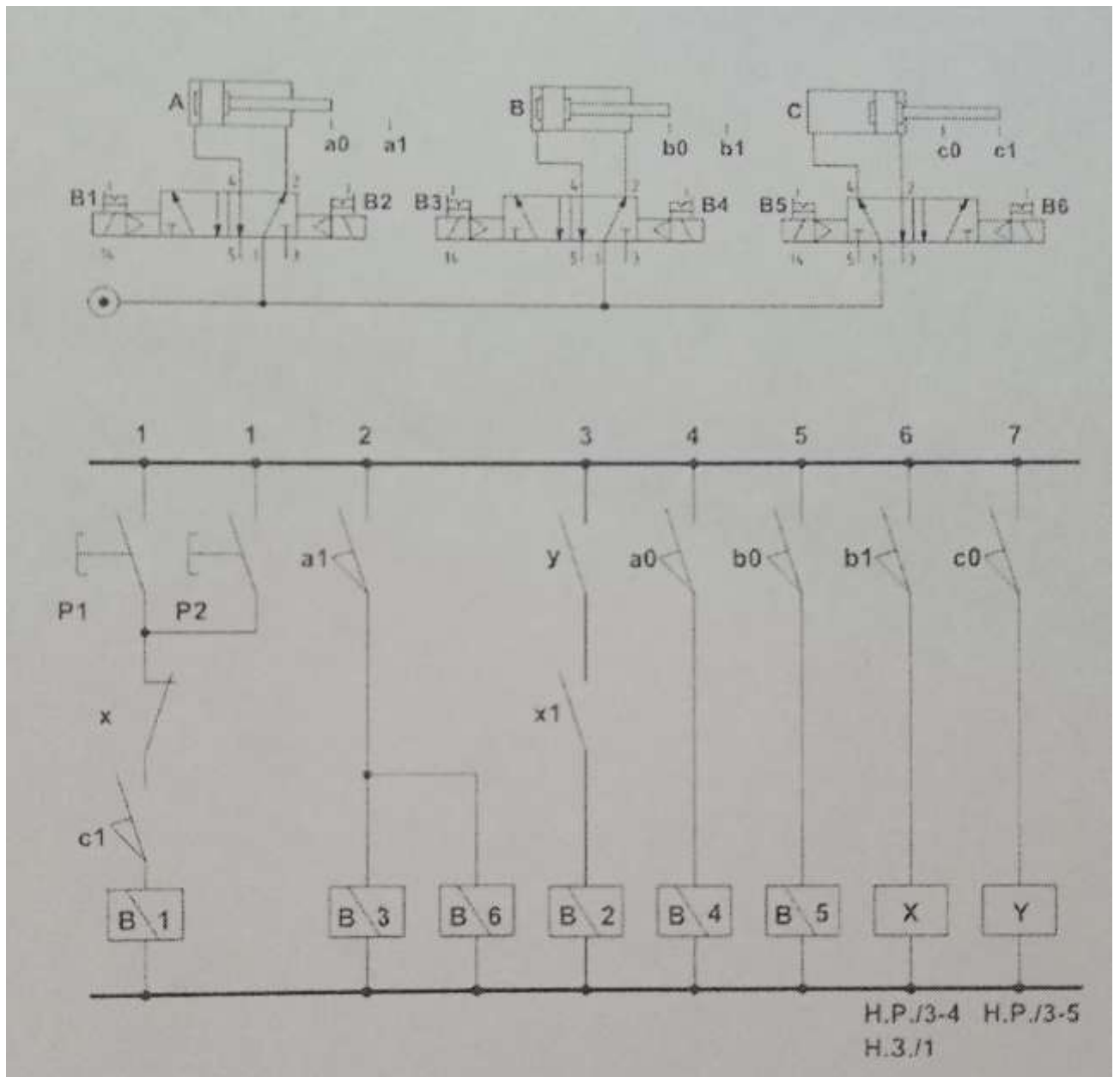
Рисунок 5 – Пневмопривод возвратно поступательного движения
