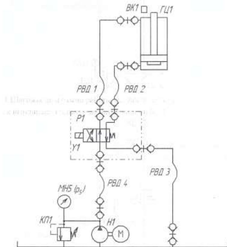
Рисунок 25.1 –Схема гидравлическая
