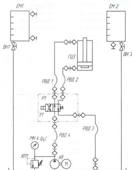
Рисунок 20.1 Схема гидравлическая
