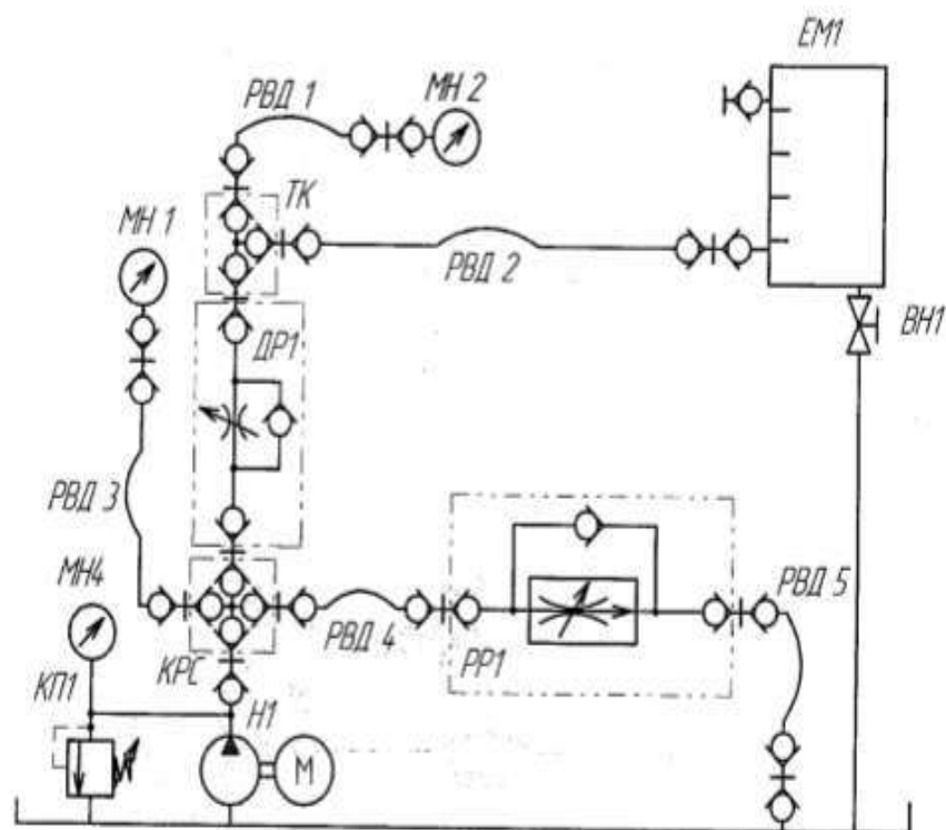
Рисунок 9– схема гидравлическая
