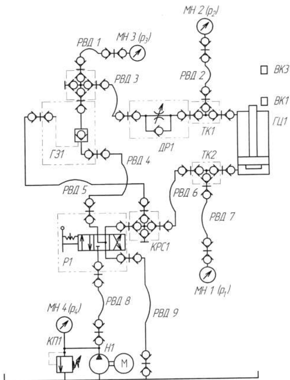
Рисунок 14.1 – схема гидравлическая
