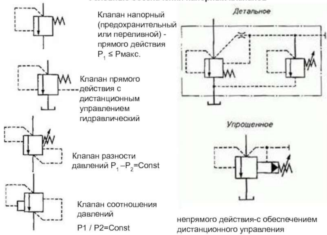
Рисунок 10.1 . Условные обозначения напорных клапанов
