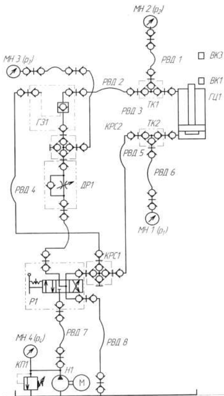
Рисунок 14.2 – схема гидравлическая
