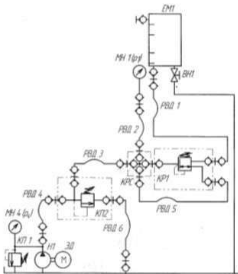
Рисунок 13.2 – схема гидравлическая
