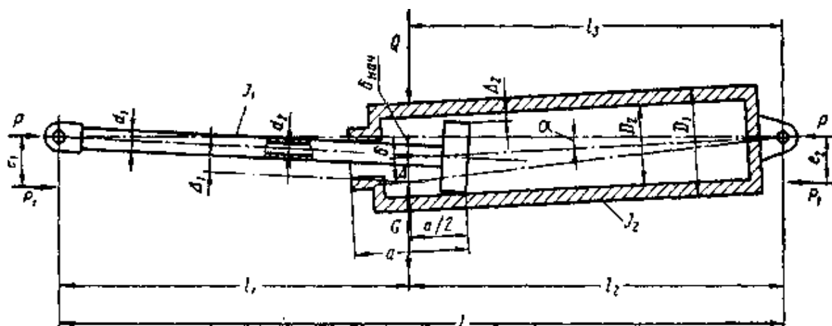
Рисунок 28.2-Схема нагружения силового цилиндра
