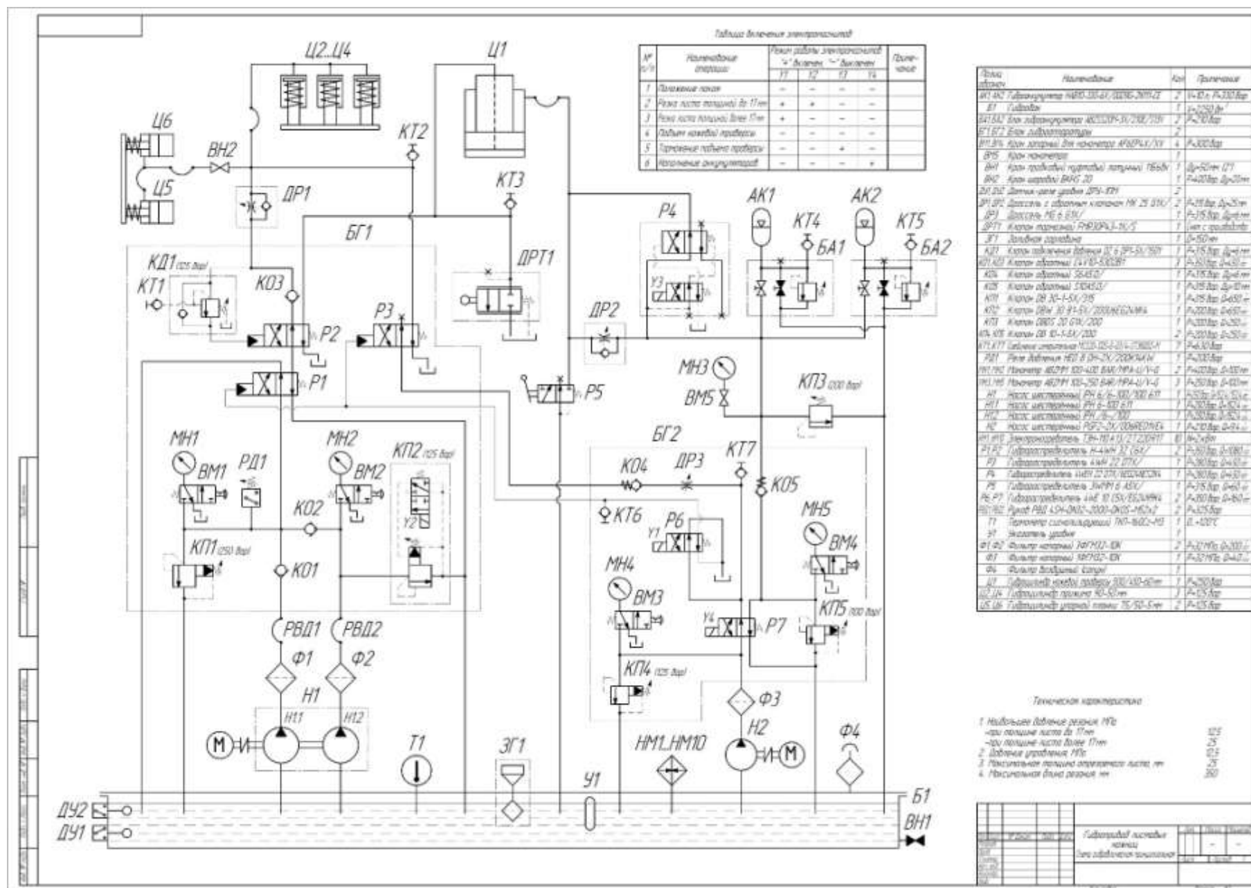
Рисунок 10.2– Гидросхема листовых ножниц
