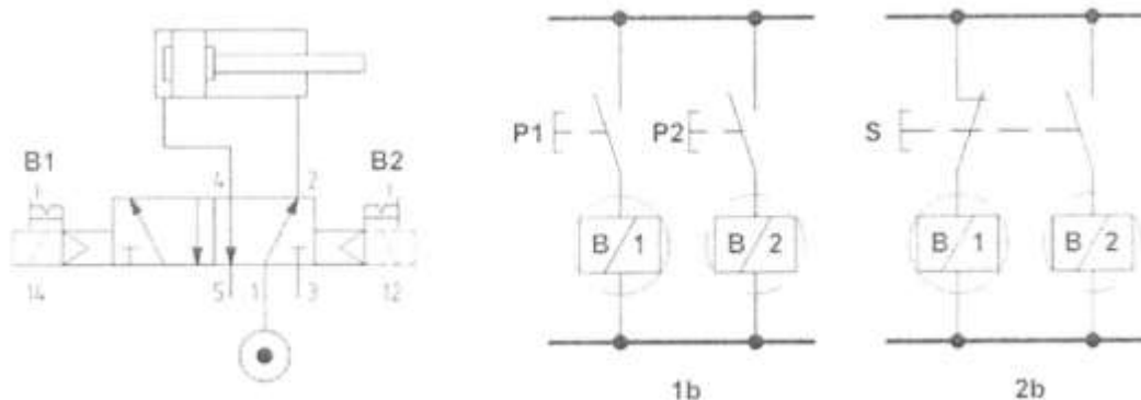
Рисунок 36 Электropневматическая схема
