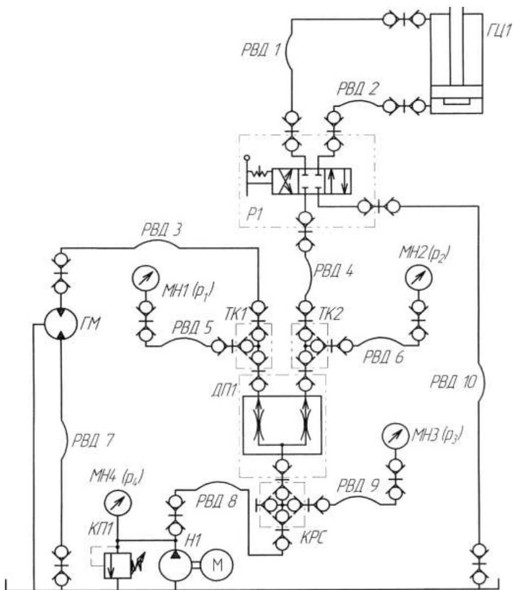
Рисунок 3 – Гидросхема гидропривода с параллельным подключением двух гидродвигателей
