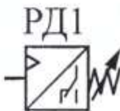
Рисунок 16.2 Обозначение датчика давления при его использовании совместно с блоком электронных реле в гидравлических схемах
