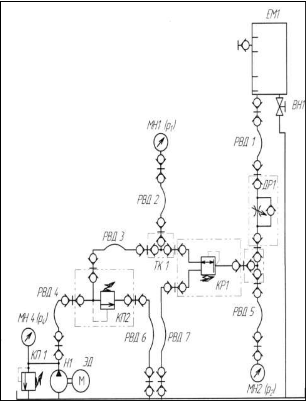
Рисунок 13.1 – схема гидравлическая
