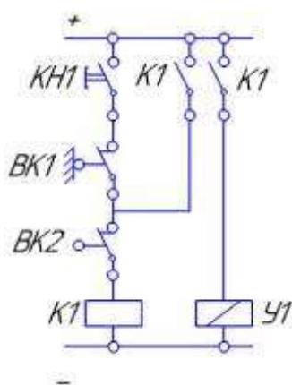
Рисунок 22.2 – Вариант 2 Изучение схем включения электро-механического датчика положения штока гидроцилиндра
