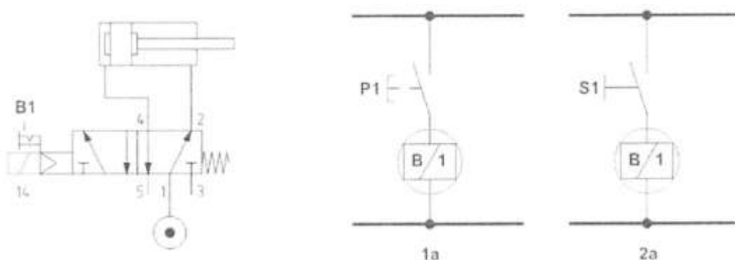
Рисунок 35 Электропневматическая схема
