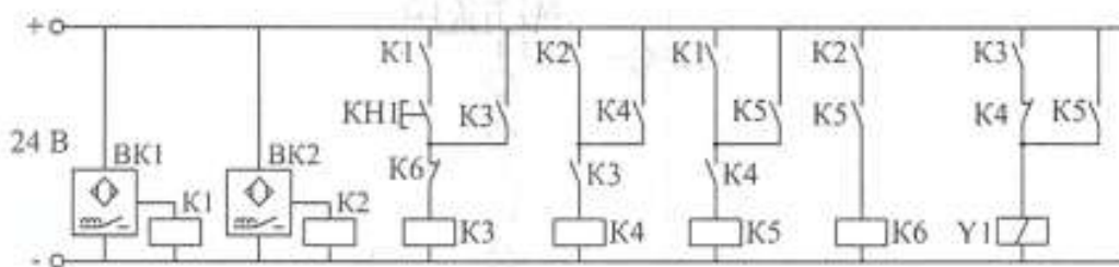
Рисунок 25.2 Схема электрическая
