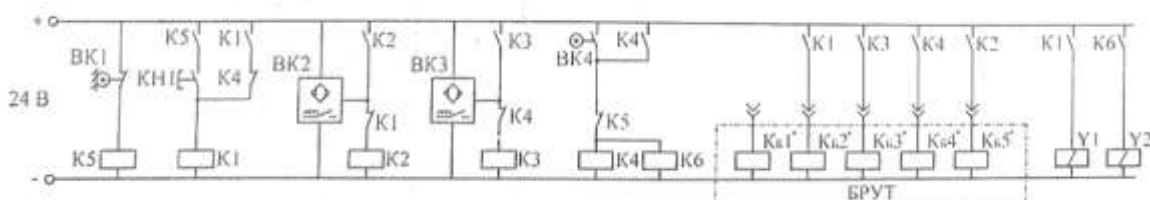
Рисунок 4 – Релейно-контактная схема
