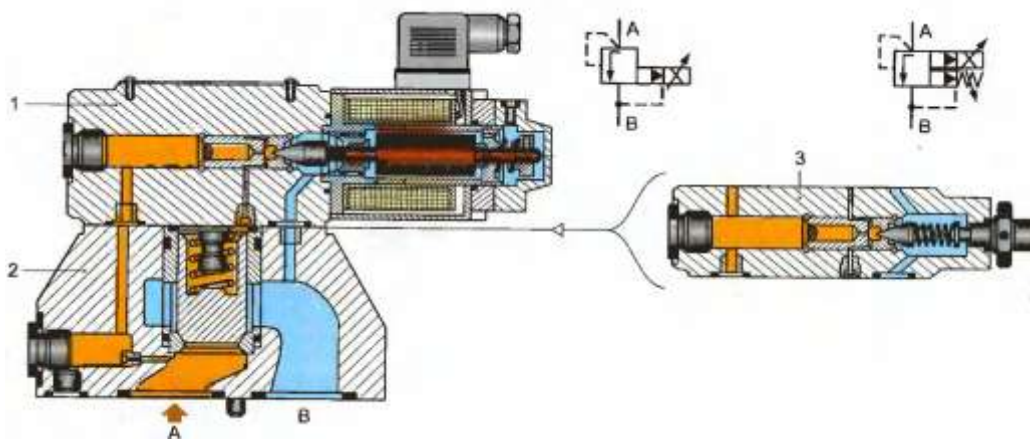
Рисунок 2 - Предохранительный клапан непрямого действия с пропорциональным управлением
