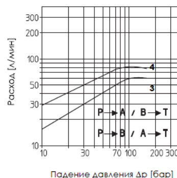
Рисунок 4 – Регулировочная характеристика распределителя
