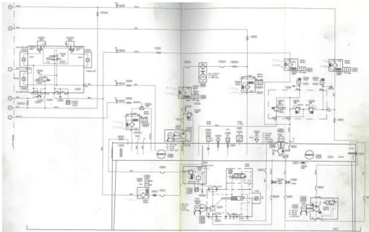
Рисунок 2 - Насосная станция.
