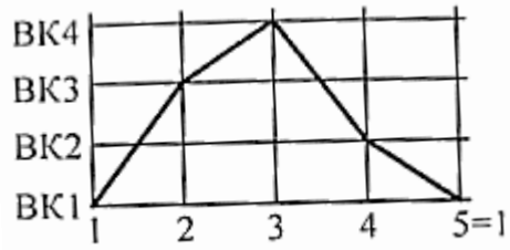
Рисунок 1 - Шаговая диаграмма работы гидравлического цилиндра.
