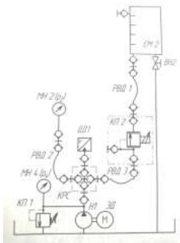
Рисунок 1 – Схема гидравлическая для выполнения лабораторной работы
