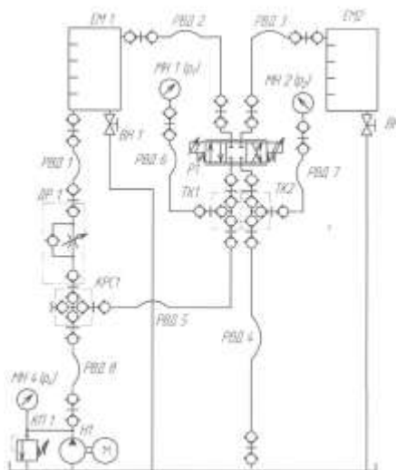
Рисунок 2 – Принципиальная гидросхема
