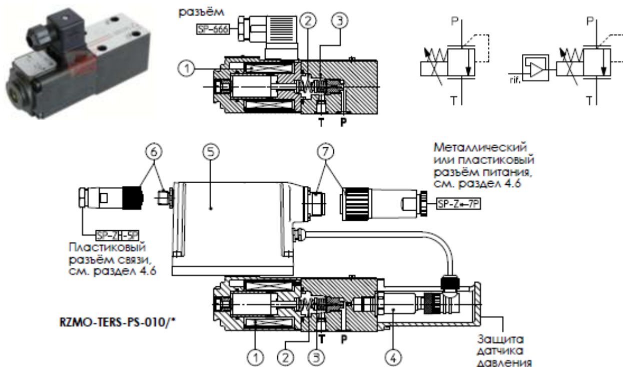
Рисунок 1 – Конструкция клапана
