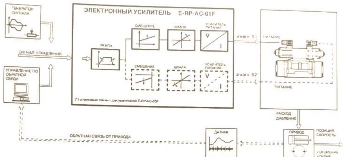
Рисунок 2 – Структурная схема использования электронного усилителя (драйвера) типа E-RP-AC-01F
