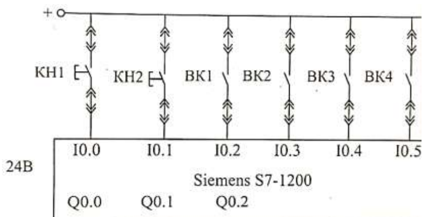
Рисунок 4 – Схема подключения ПЛК
