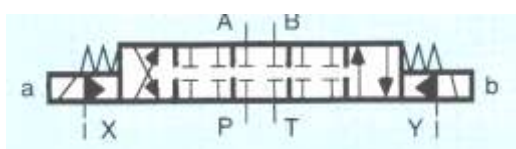
Рисунок 2 - Переходные положения золотника обычного и пропорционального распределителей с одинаковой схемой исполнения
