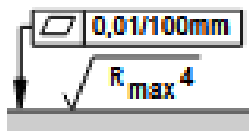
Рисунок 2 - Требования к сопрягаемой поверхности
