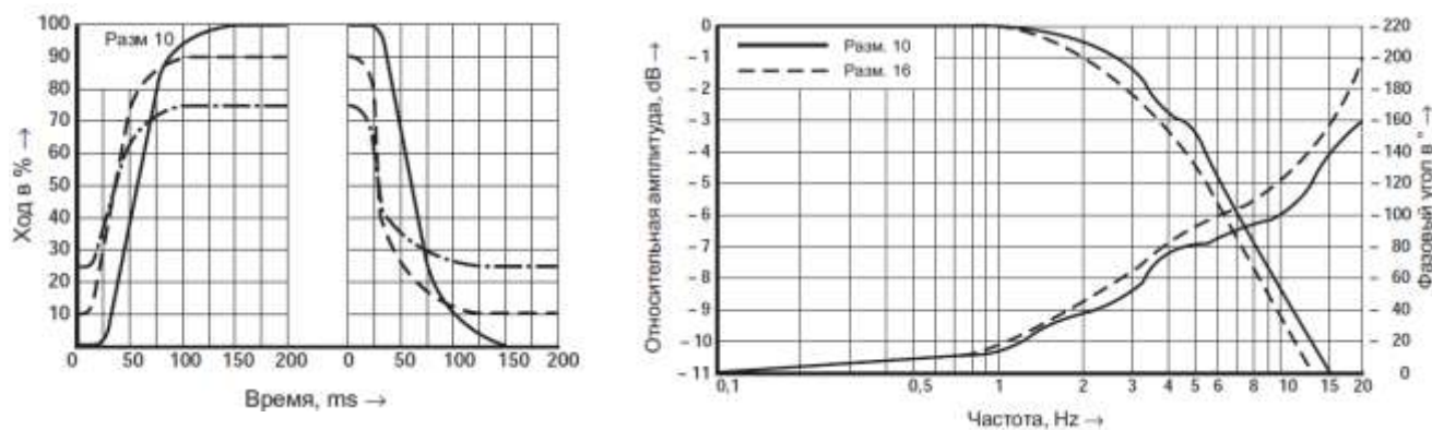
Рисунок 2 – Переходной процесс при ступенчатом входном сигнале и амплитудно-частотная характеристика
