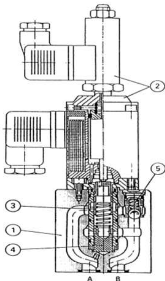
1 - корпус; 2 - управляющий электромагнит с индуктивным датчиком перемещения якоря; 3 - измерительная диафрагма; 4 - клапан постоянной разности давлений; 5 - обратный клапан; А, В - присоединительные отверстия
