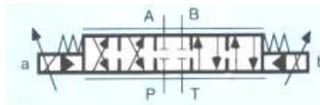
Рисунок 2 - Переходные положения золотника обычного и пропорционального распределителей с одинаковой схемой исполнения
