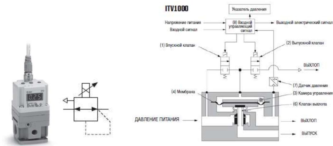
Рисунок 1 - Принципиальная схема
