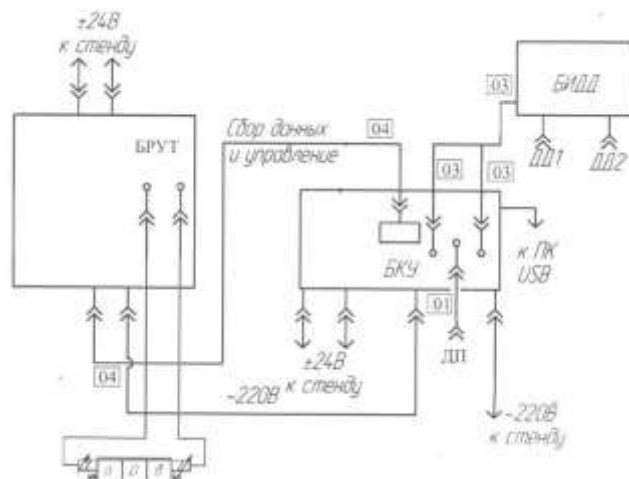
Рисунок 2 – Принципиальная электросхема
