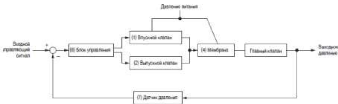
Рисунок 2 – Структурная схема
