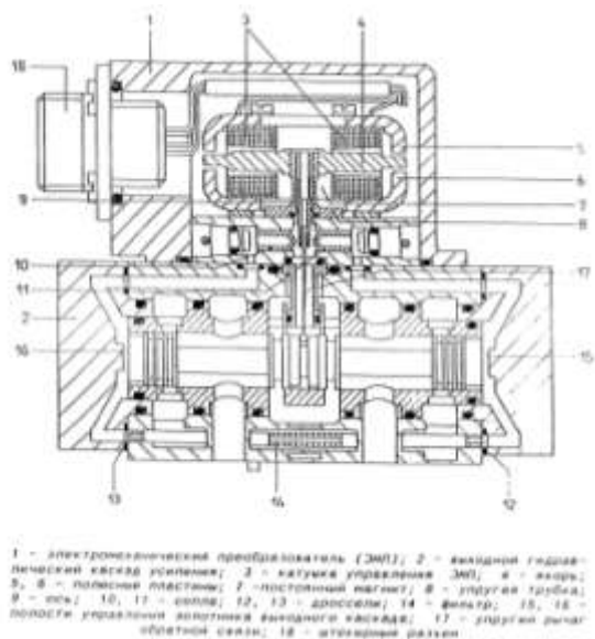
Рисунок 1 - Двухкаскадный электрогидравлический усилитель с механической силовой обратной связью
