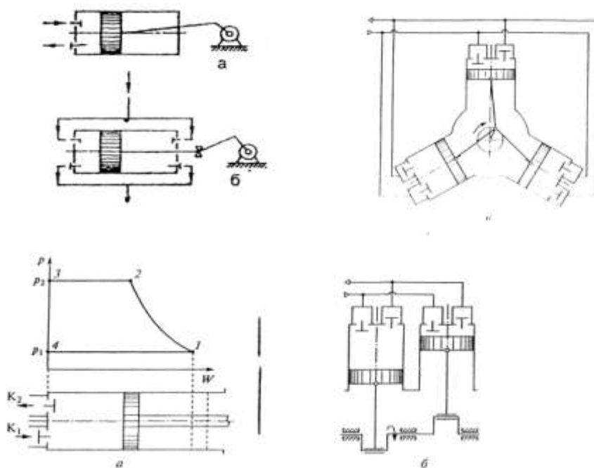
Рисунок 1 - Схемы поршневых компрессоров: а - одноступенчатого одностороннего действия; б - двуступенчатого двустороннего действия
