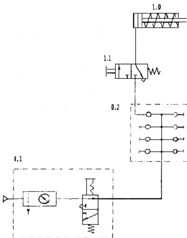
Рисунок 1 - Принципиальная схема
