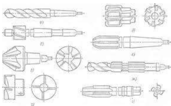
Рисунок 1. Стандартизованные приспособления
