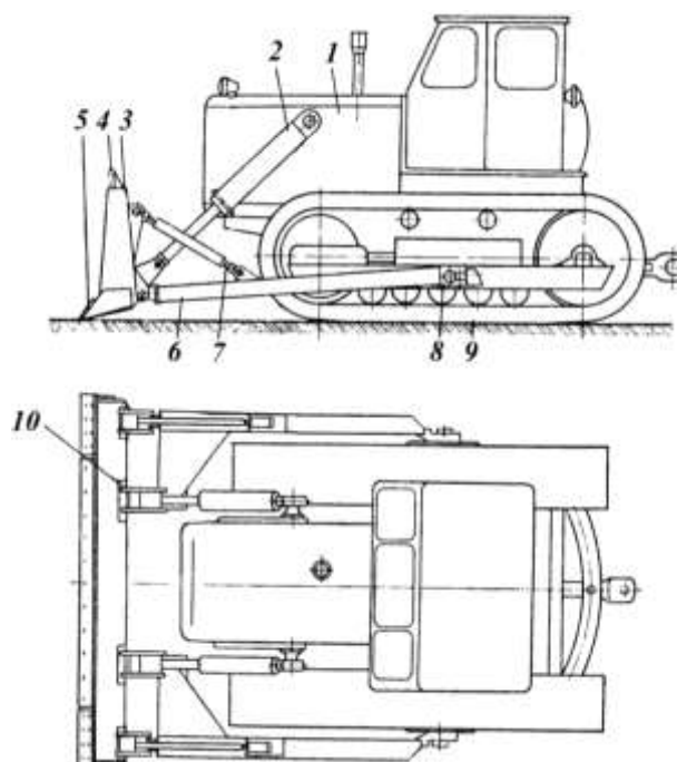
Рисунок 1.1 - Устройство бульдозера с неповоротным отвалом:
