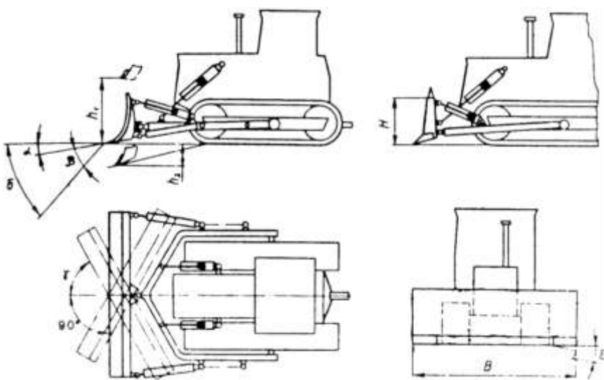
- Основные параметры бульдозерного оборудования
