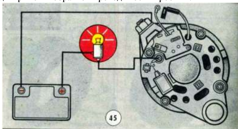
Рисунок 19 Проверка диодов выпрямительного блока на пробой на автомобиле 12.2 Проверьте диоды прямой проводимости
