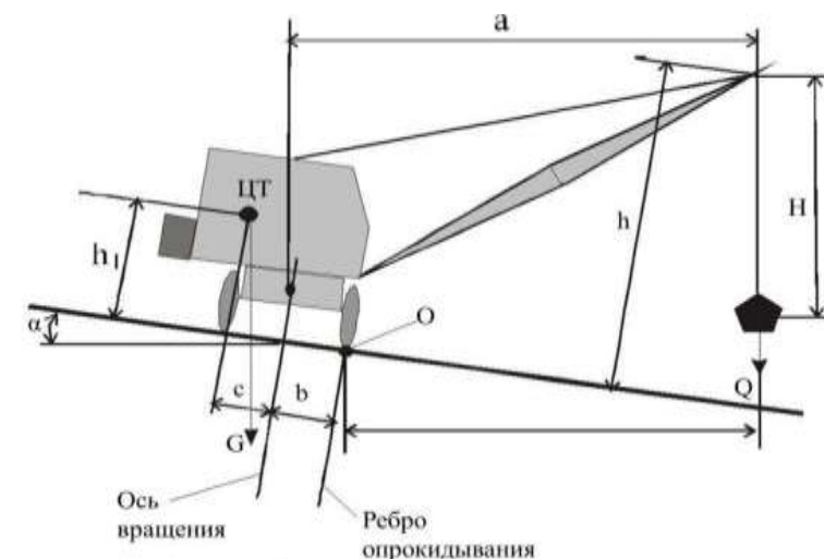
Рисунок 5. Расчетная схема грузовой устойчивости крана с грузом
