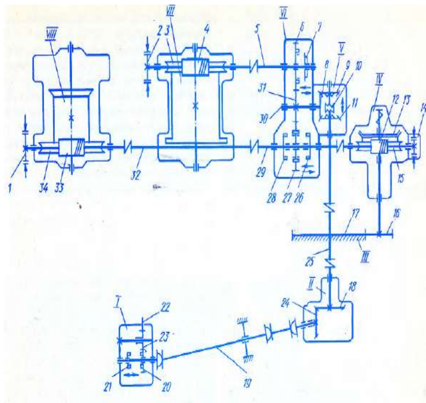
Рис. 58. Кинематическая схема кранов КС-2561Д:
