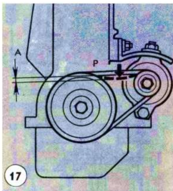
Рисунок 4. Проверка натяжения ремня привода генератора
