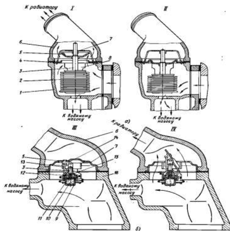
6. Принцип работы гидромуфты двигателя КамАЗ - 740.
