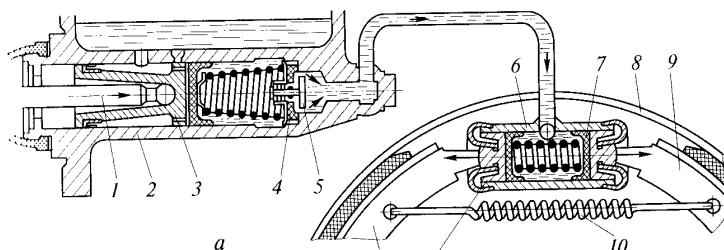
Рис.17.1 Схема тормозного механизма с гидравлическим приводом:
