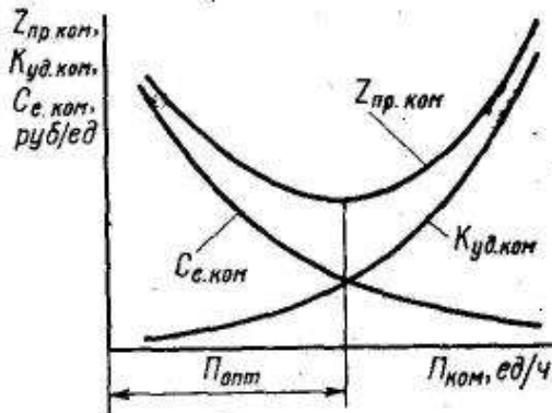
Рис. 4 Функциональная зависимость производительности комплекса P_{ком} машин от себестоимости единицы его продукции С_{е.ком} , удельных капиталовложений К_{уд.ком} и приведенных затрат Z_{пр.ком}
