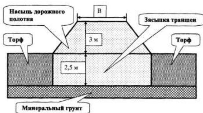
Рис. 1. Расчетная схема выторфовывания болота
