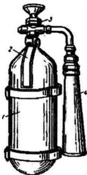
Рис. 2. Огнетушитель ОУ-2:
